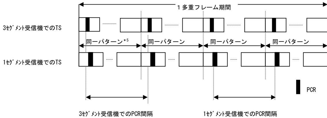
図3.4.1-4 Mode3でのPCRパッケージ伝送
