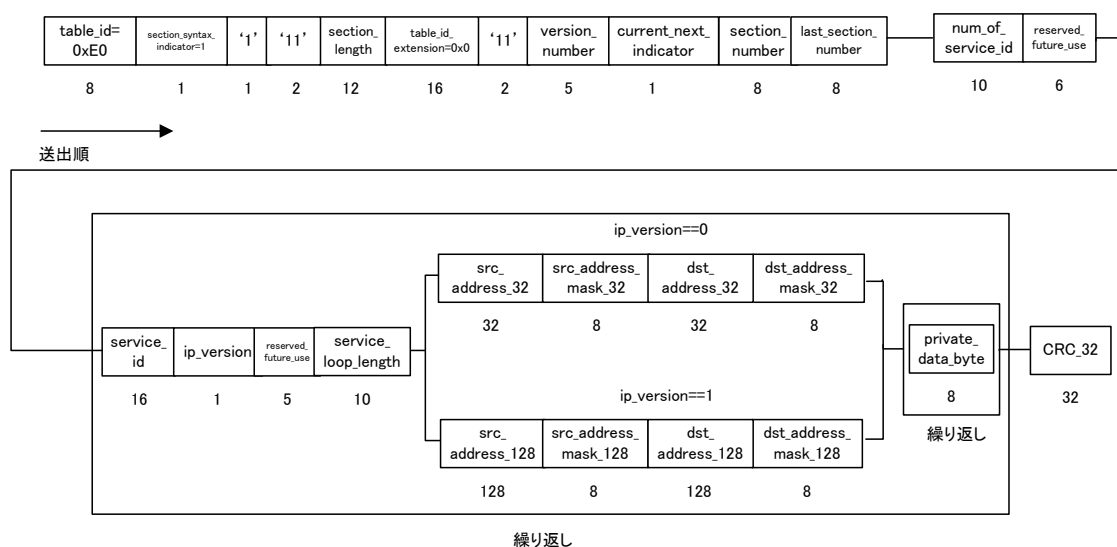
図3.4.3.3.1-1 AMTの構成
