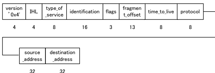
図3.4.3.2.1-2 IPv4_header_wo_length( )の構成
