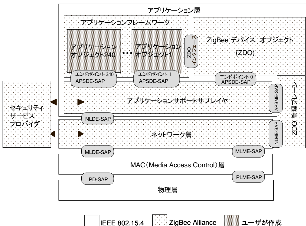
図 2.2-1 ZigBee のプロトコル構成
