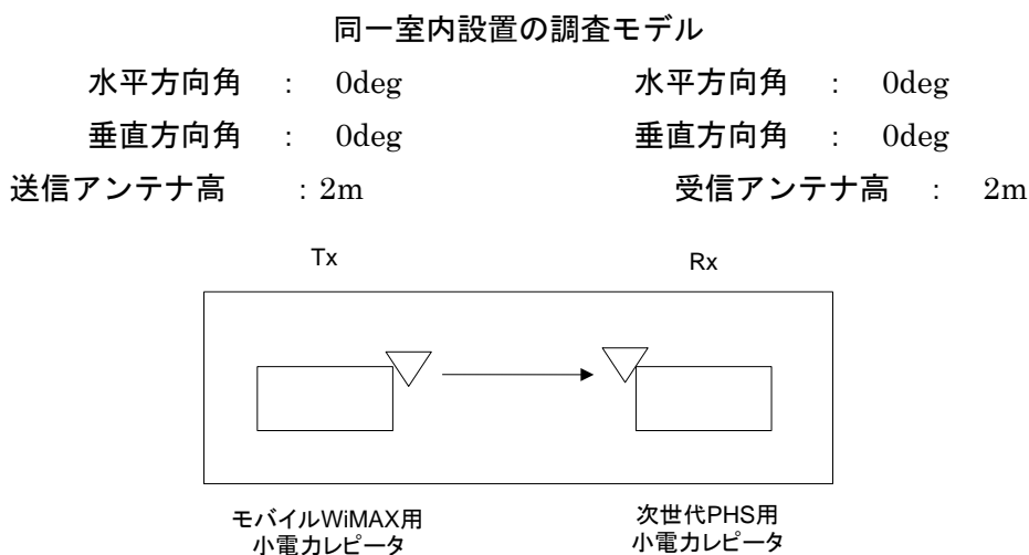
図2.6-1 同一室内設置の調査モデル
