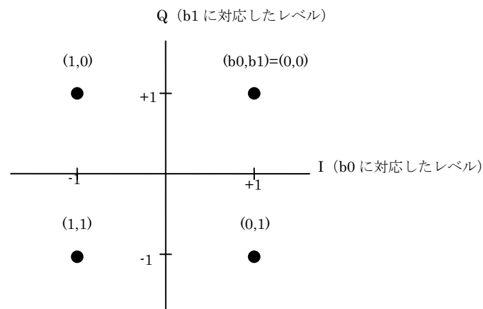
図 3.1.6.9-5 QPSK 位相図
