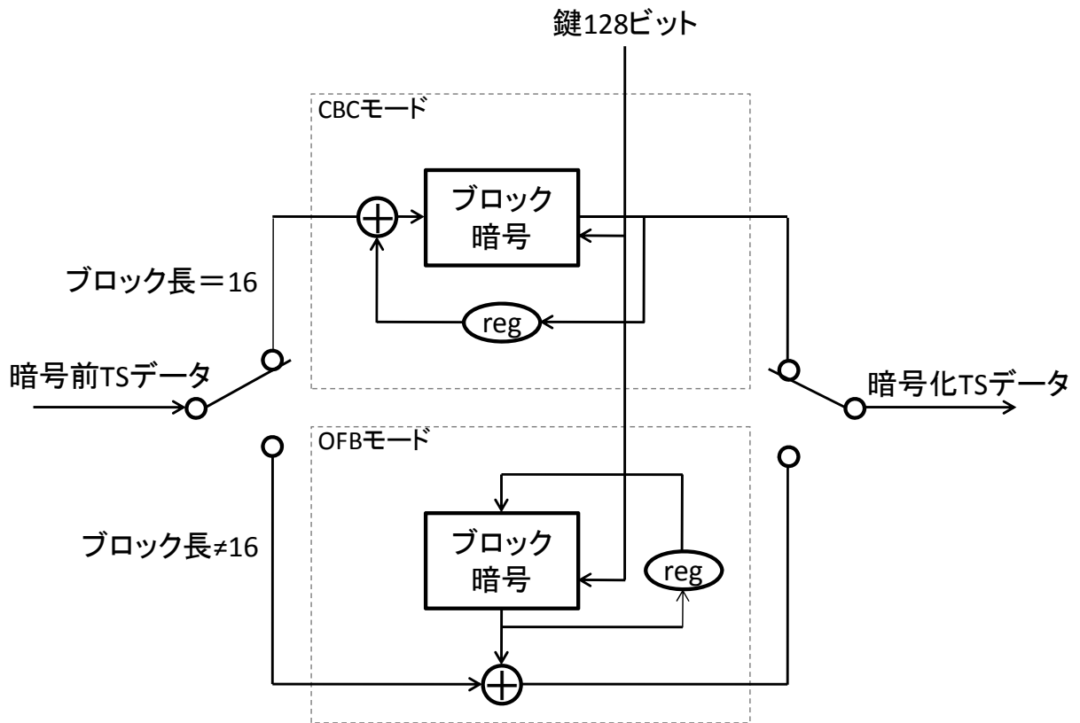
図 3.1.4.2-1 スクランプル方式は、128ビットブロック暗号を適用した場合の例である。
