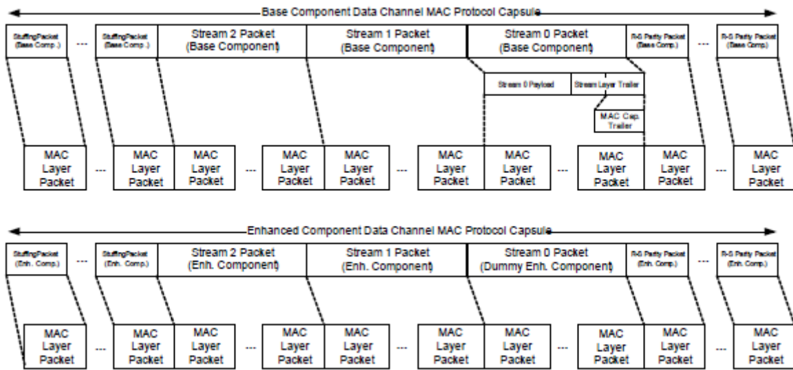
図3.2.5.5-2 データチャンネルMACプロトコルのカプセル化 (レイヤード)
