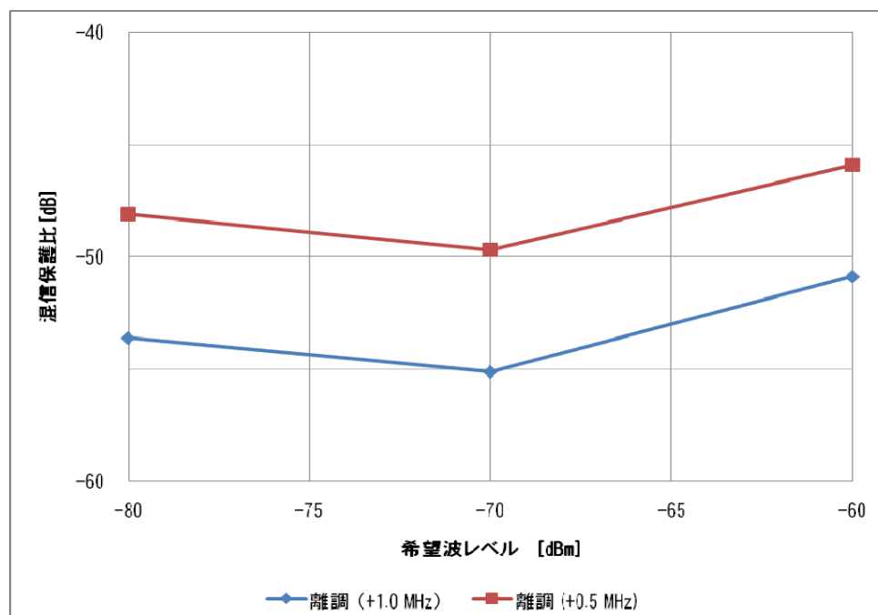
図 3.2.7.4.1.1-4 希望波入力レベル対 ESR 所要 DU (MediaFLO (上隣接) to MediaFLO)
