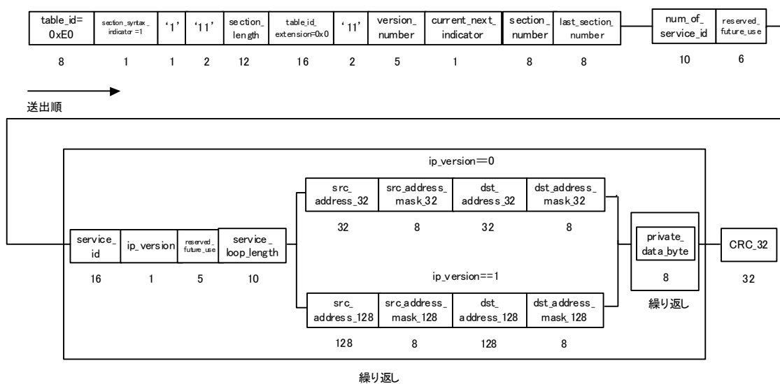
図3. 3. 5. 4. 3. 1-1 AMTの構成
