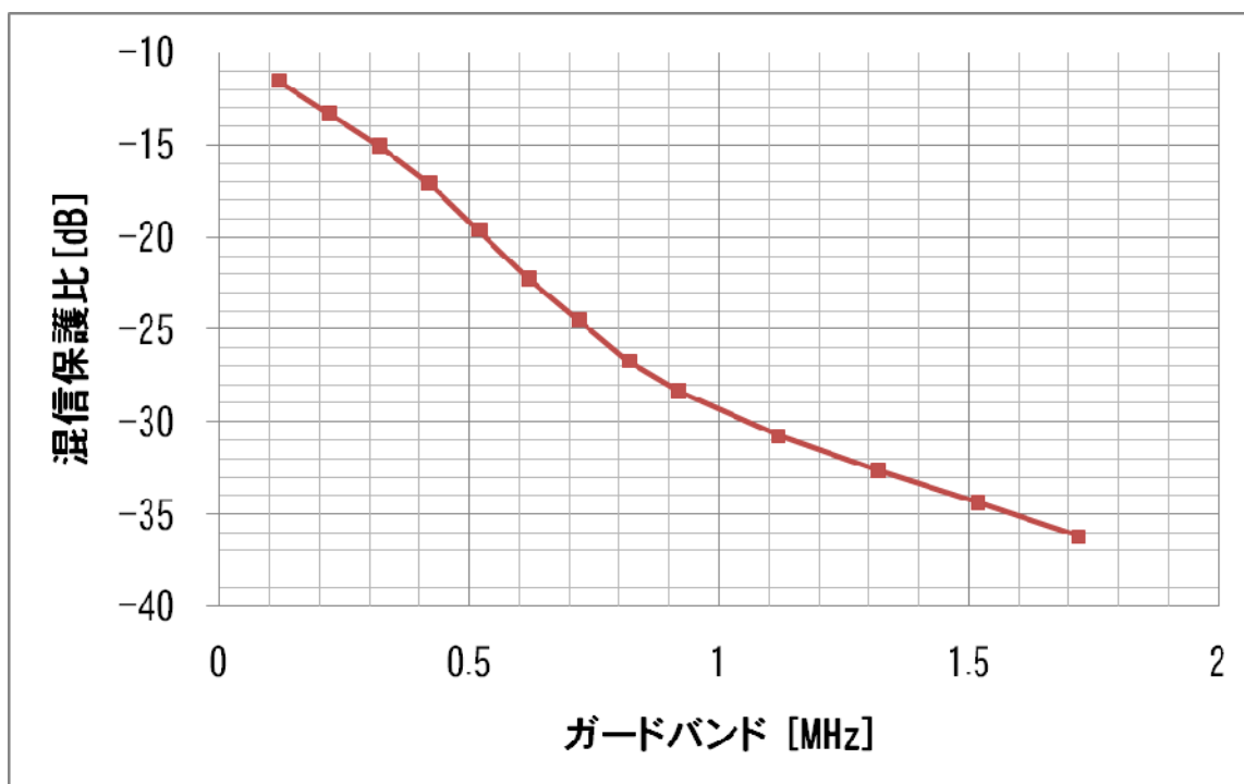
図 3.2.7.4.1-3(b) ガードバンド対混信保護比 (ISDB-Tmm to MediaFLO)
