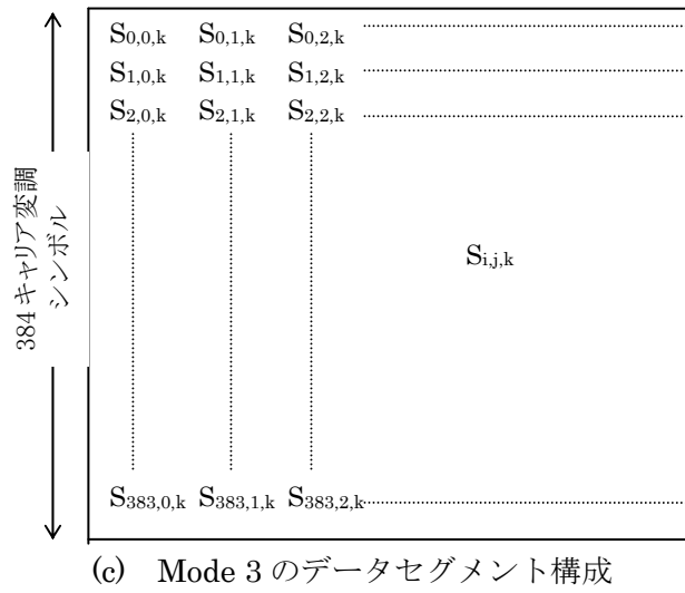
図 3.1.6.9-10 データセグメントの構成
