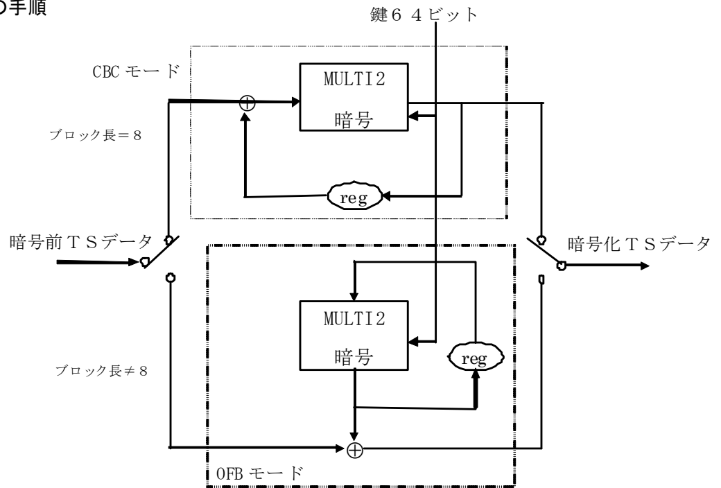
図 3.3.4.1.1-1 スクラブル方式
