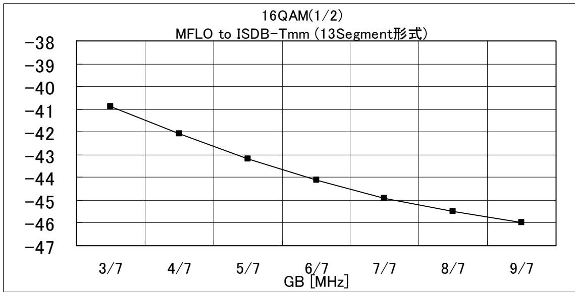
図 3.1.8.4-7 5%ESR 所要 DU 対ガードバンド (MFLO to ISDB-Tmm (13 セグメント形式))
