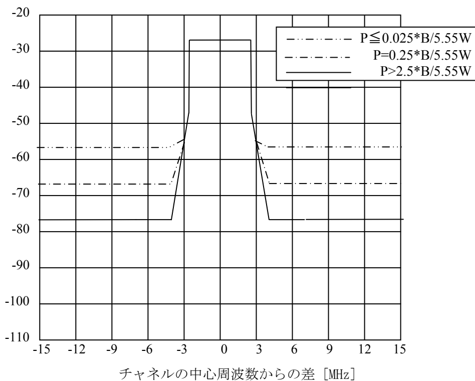
図 3.2.2.5-1 MediaFLO 方式マルチメディア放送の送信スペクトルマスク ( B=4.625 、 6.475 もしくは 7.4\text{MHz} )
