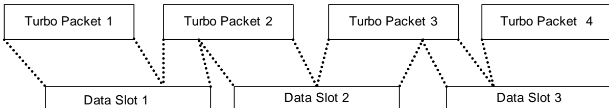
図3.2.6.20.5-4 ベースおよびエンハンスメントコンポーネントの交互配置
