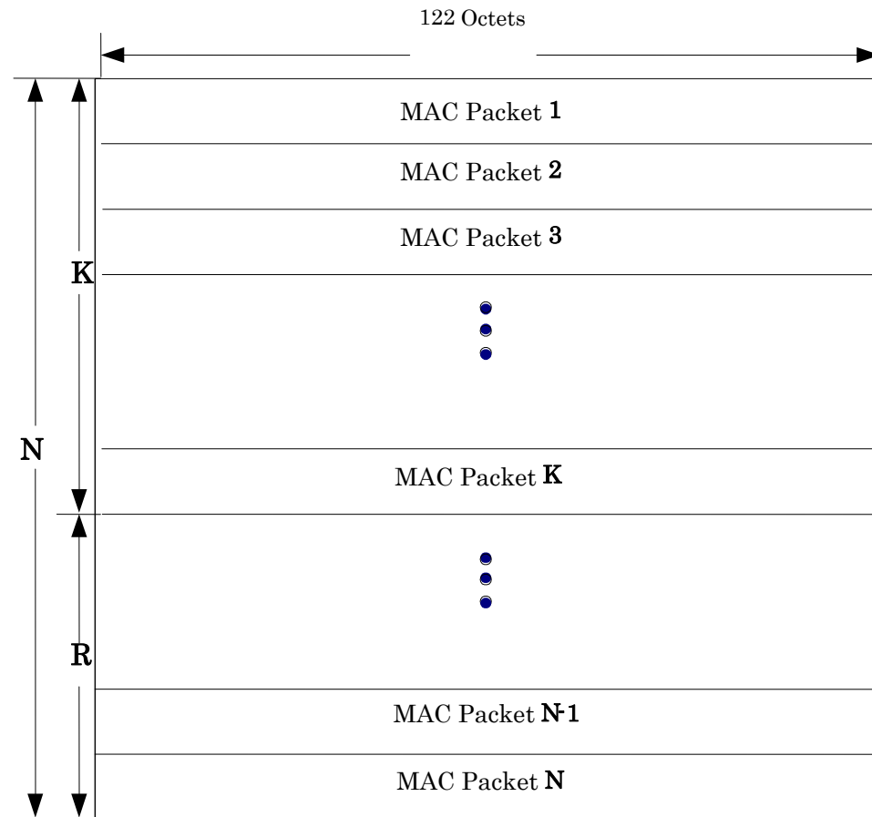
図 3.2.6.24-1 ラプター誤り制御ブロック構成
