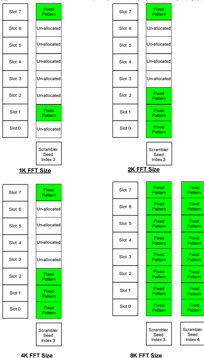
図3.2.6.12.1-1 TDMパイロット2チャンネルスロット割り当て
