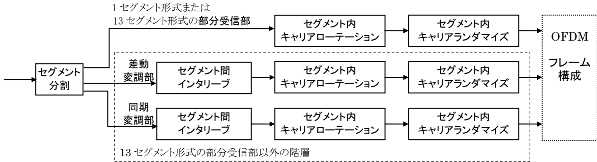
図 3.1.6.11-3 周波数インタリーブの構成
