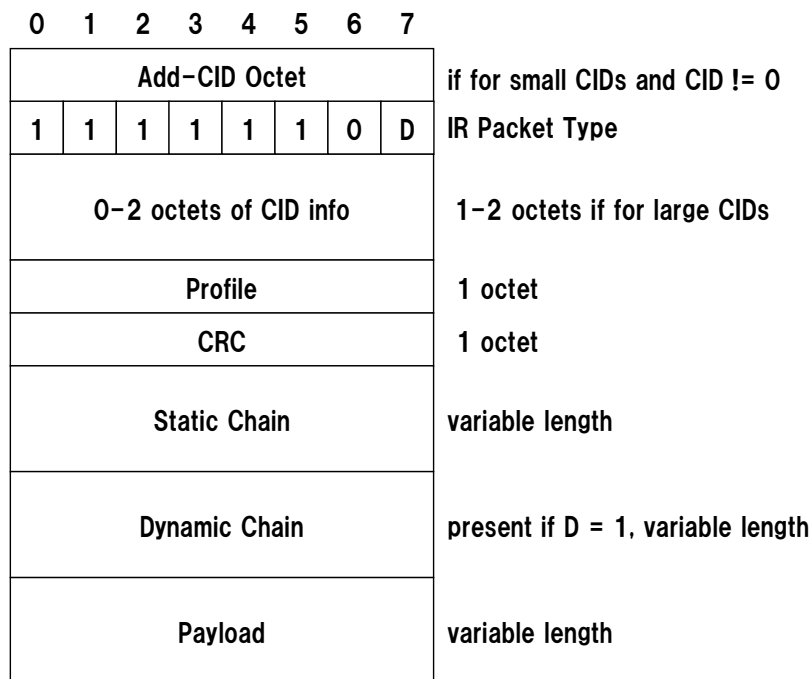
図 3.1.5.4-34 IR パケット構造
