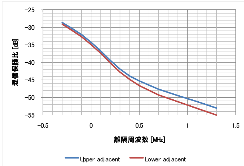
図 3.2.7.4.1.1-2 5%ESR 所要 DU 対離隔周波数 (ISDB-Tmm to MediaFLO)
