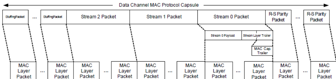
図3.2.5.5-1 データチャンネルMACプロトコルのカプセル化 (ノンレイヤード)
