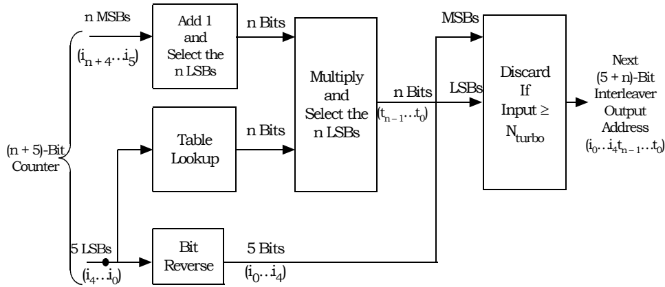
図 3.2.6.16.1.2-1 ターボインターリーバーの出力アドレス計算処理
