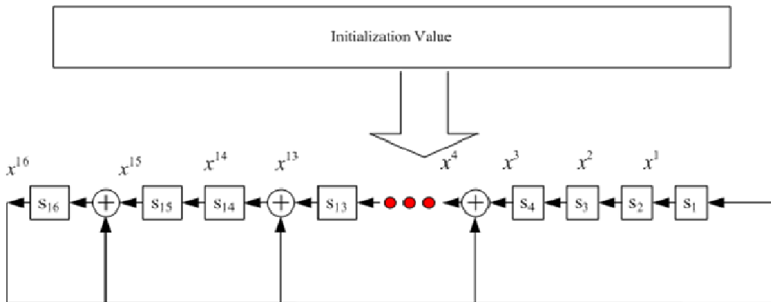
図3.2.6.20.3-2 Mシーケンスインターリーバー (16-bit)
