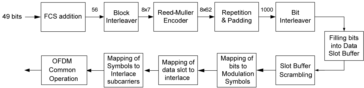
図3.2.6.14.2.3-1 スロット3の処理
