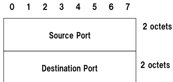
図 3.1.5.4-42 UDP ヘッダ (Static Part)
