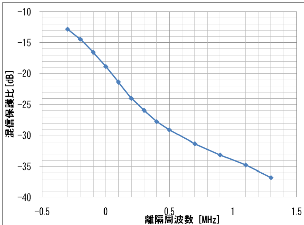
図 3.2.7.4.1-2(a) 離隔周波数対混信保護比 (MediaFLO to MediaFLO)
