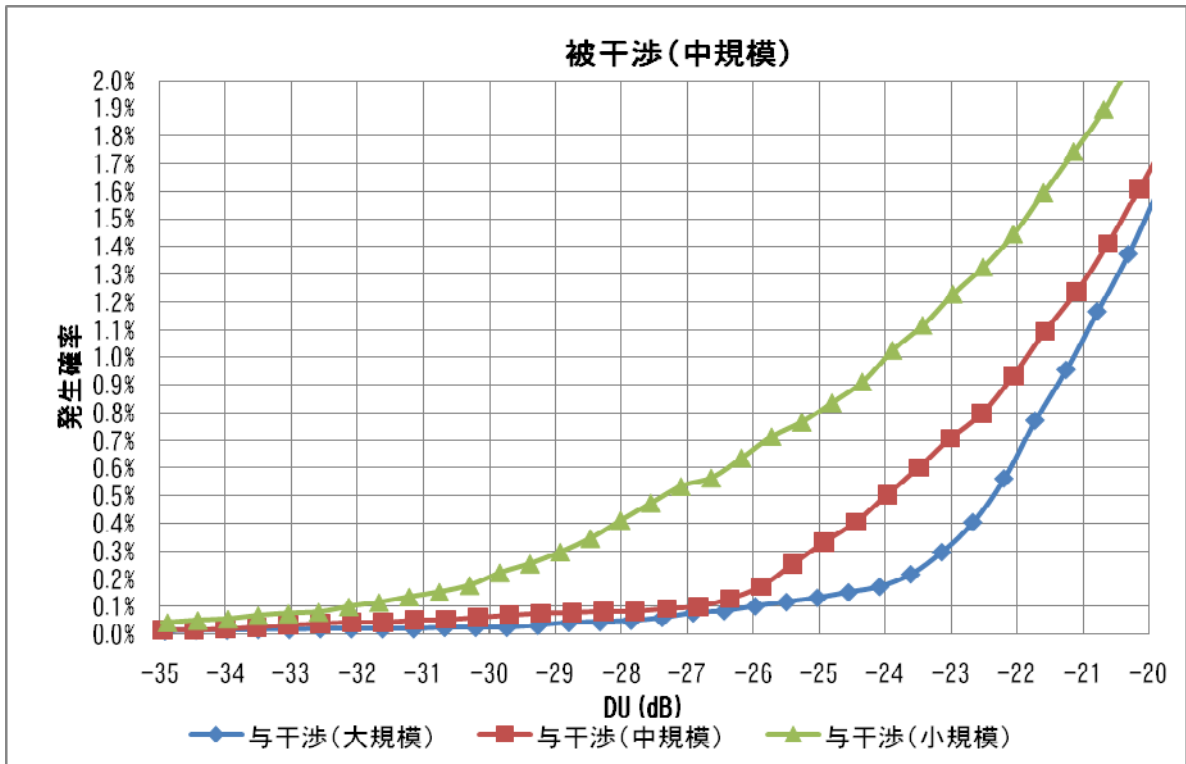
図 3.2.7.4.2.1-4 中規模局（被干渉）の DU 分布
