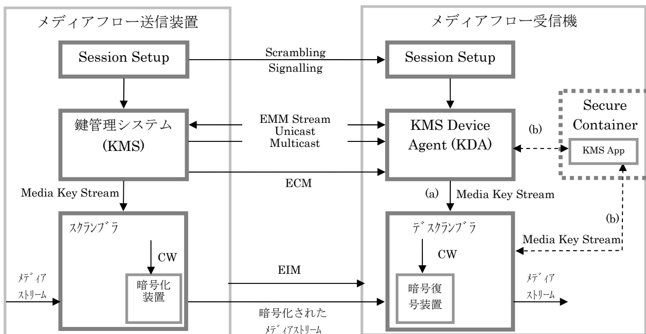
図 3.2.4.2-1 限定受信方式のアーキテクチャ
