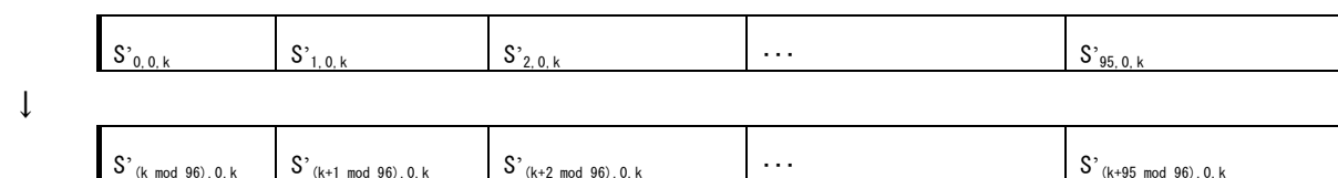
図3.3.6.11.2.2-1(a) Mode 1のキャリアローテーション
