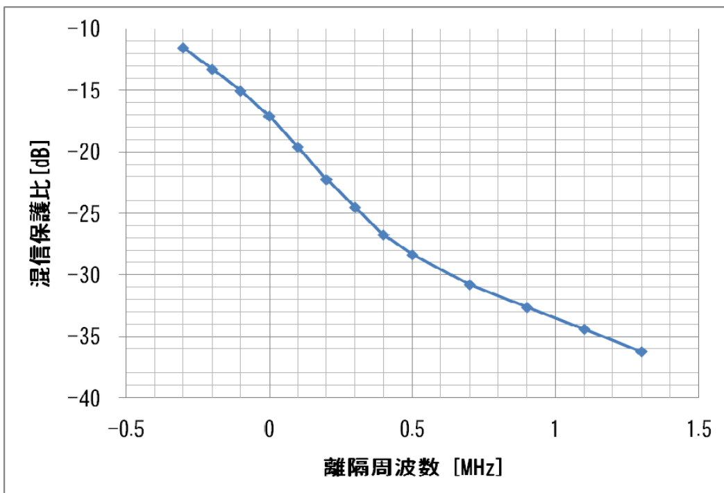
図 3.2.7.4.1-3(a) 離隔周波数対混信保護比 (ISDB-Tmm to MediaFLO)
