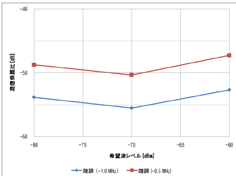
図 3.2.7.4.1.1-3 希望波入力レベル対 ESR 所要 DU (MediaFLO (下隣接) to MediaFLO)
