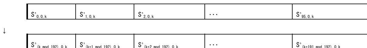
図3.3.6.11.2.2-1(b) Mode 2のキャリアローテーション
