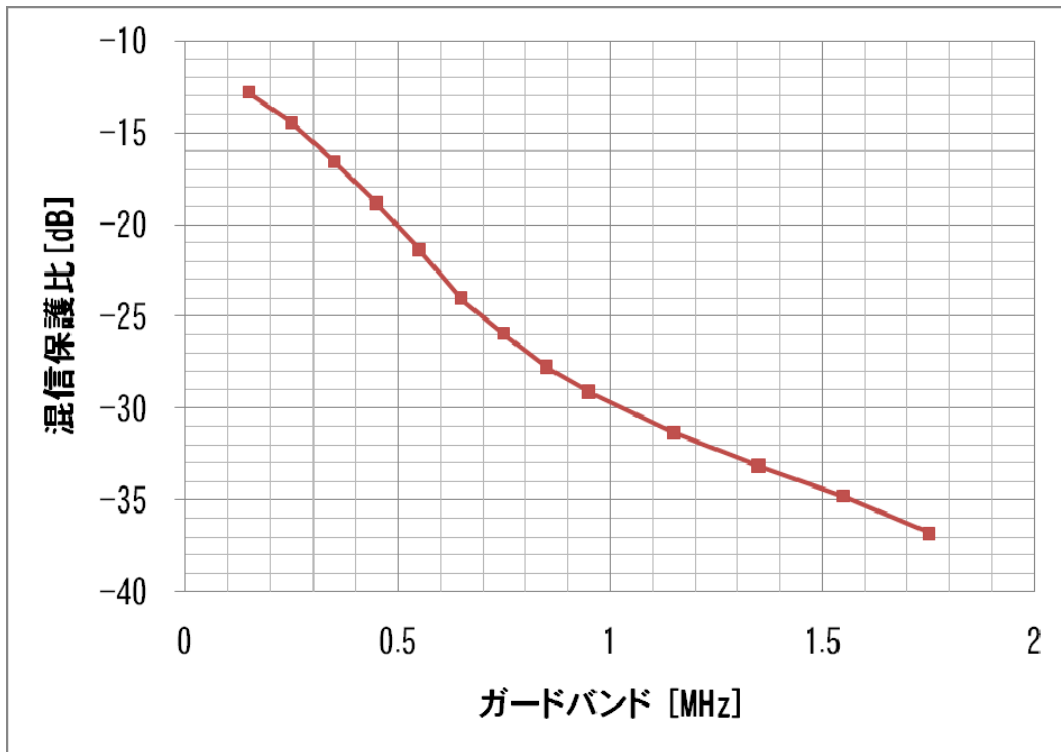
図 3.2.7.4.1-2(b) ガードバンド対混信保護比 (MediaFLO to MediaFLO)
