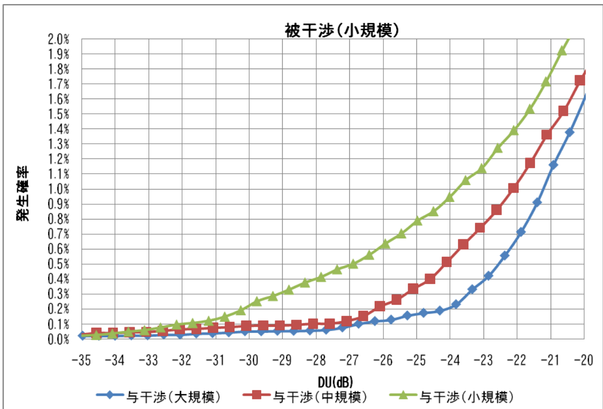
図 3.2.7.4.2.1-5 小規模局（被干渉）の DU 分布
