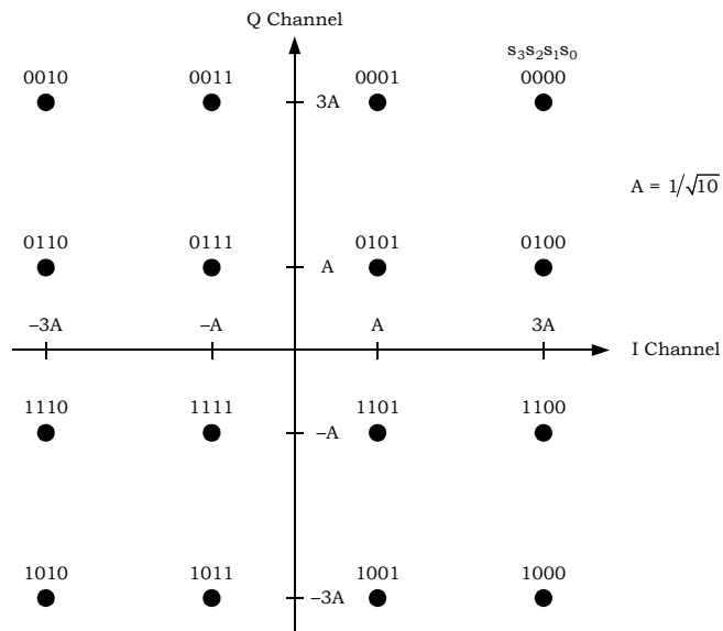
図 3. 2. 6. 20. 7. 2-1 16QAM 位相図
