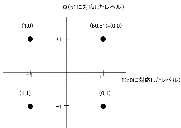
図3.3.6.9.2.1-2 QPSK位相図
