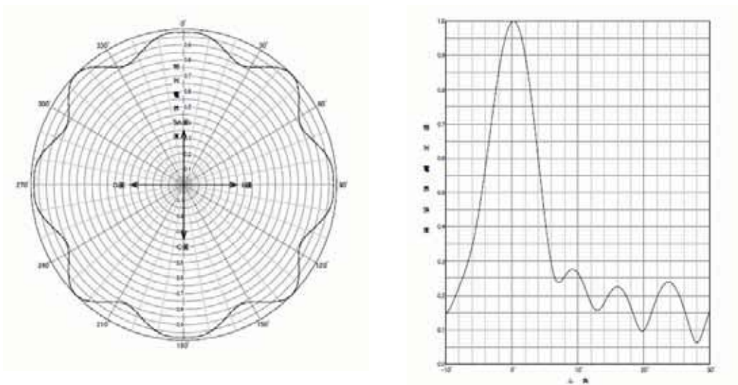
図 3.2.7.4.2.1-1 大規模基地局のアンテナパターン (2 ダイポール 8 段 4 面)
