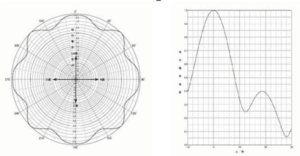
図 3.2.7.4.2.1-2 中規模基地局のアンテナパターン (2 ダイポール 4 段 4 面)
