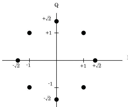
図 3.1.6.9-3 \pi/4 シフト DQPSK 位相図
