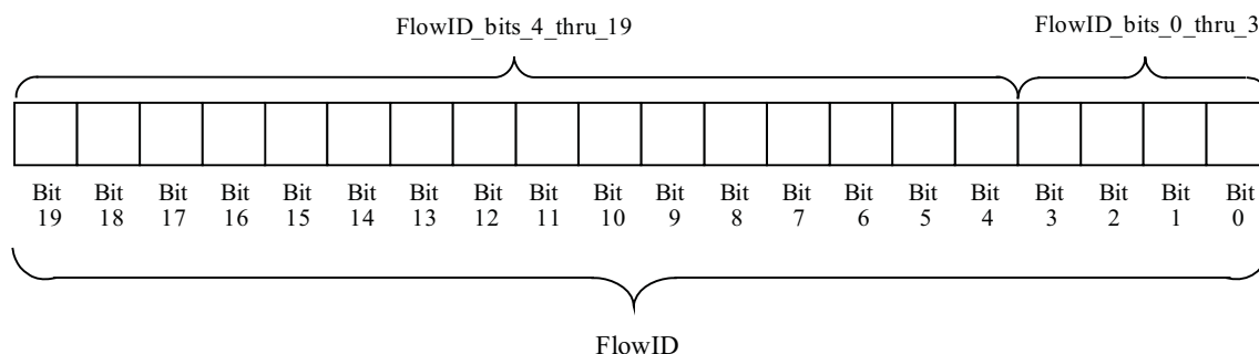
図 3.2.6.25-1. FlowID 構造
