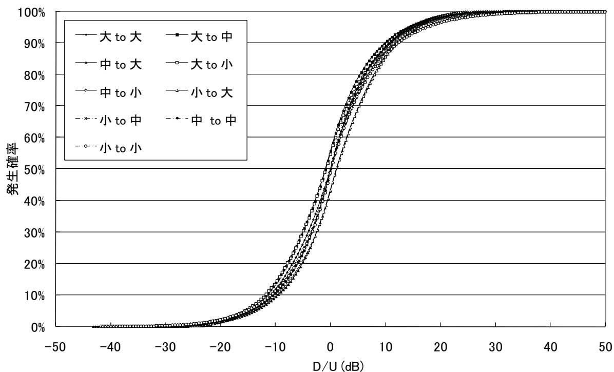
図 3.2.7.4.2.1-6 D/U 分布図全体
