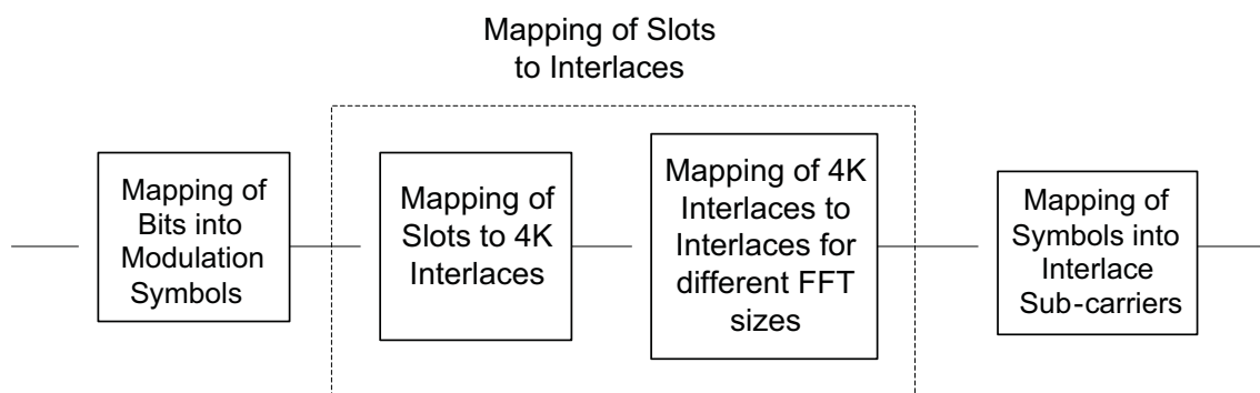
図3.2.6.12.5-1 TDMパイロット2チャンネル スロット・インターレースマッピング
