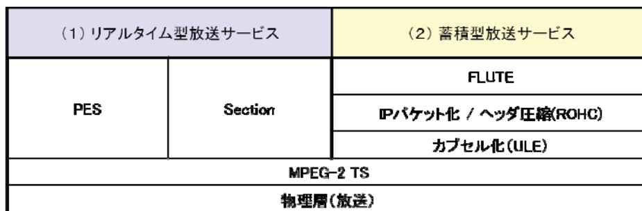
図 3.1.5.1-1 ISDB-Tmm のプロトコルスタック
