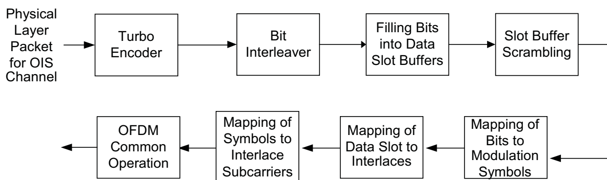
図3.2.6.16-1 OISチャンネルの処理ブロック
