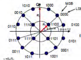
図10 16APSK ビットマッピング
