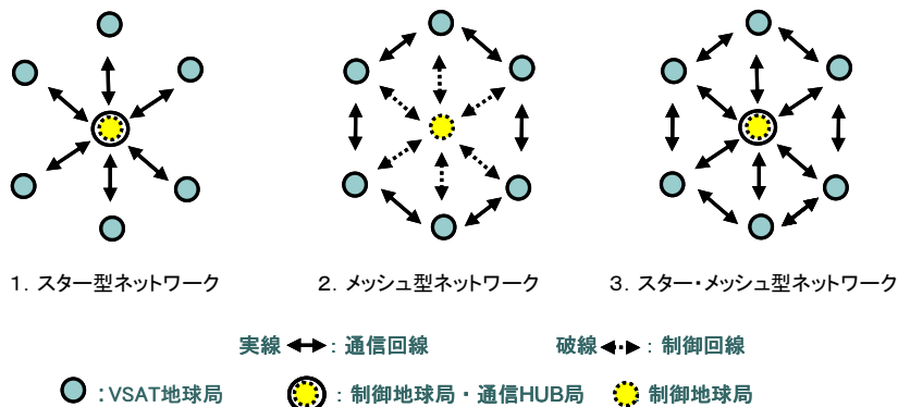
図2-2:VSAT ネットワーク構成
