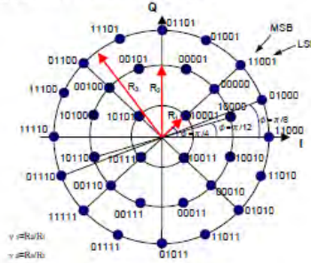
図11 32APSK ビットマッピング
