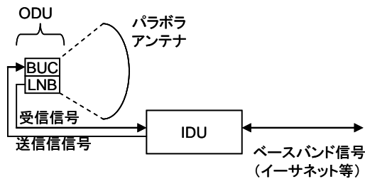
図2-3 VSAT 地球局の構成
