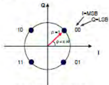
図8 QPSK ビットマッピング
