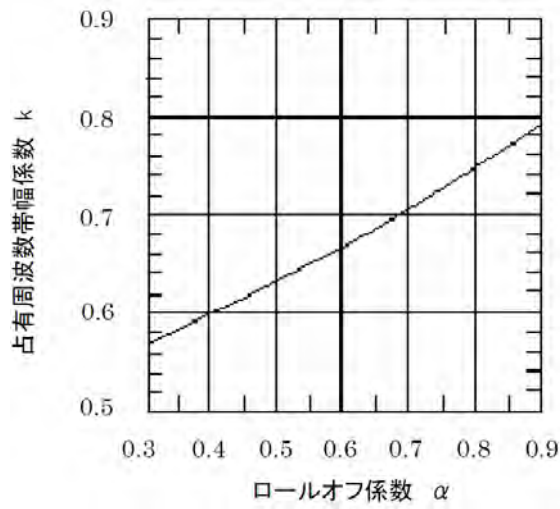
図2 占有周波数帯幅係数 k
