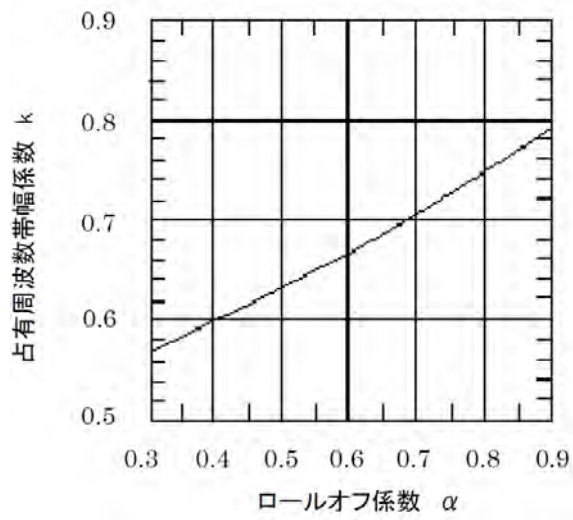
図3-2 占有周波数帯幅係数 k
