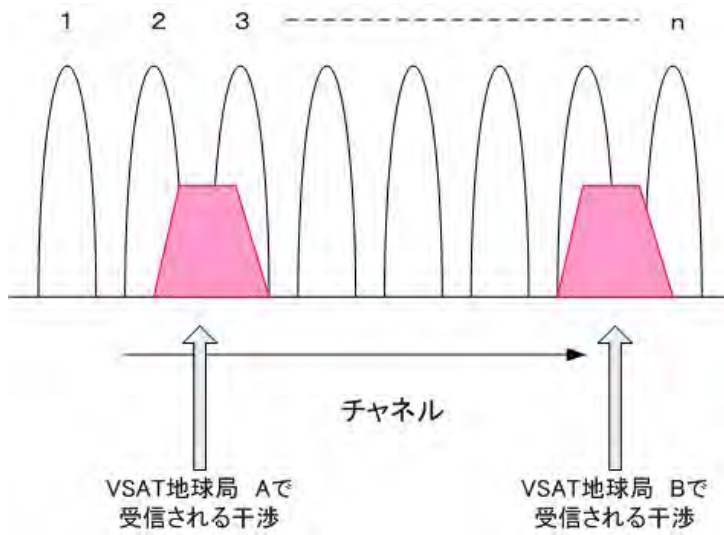
別図3 周波数割当てでの干渉回避
