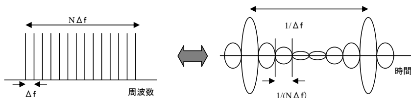
図2-1a : 周波数軸上のCI信号群
