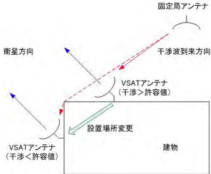
別図1 ベランダ設置の場合の設置場所変更による干渉回避
