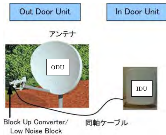
図2 VSAT 地球局の構成例
