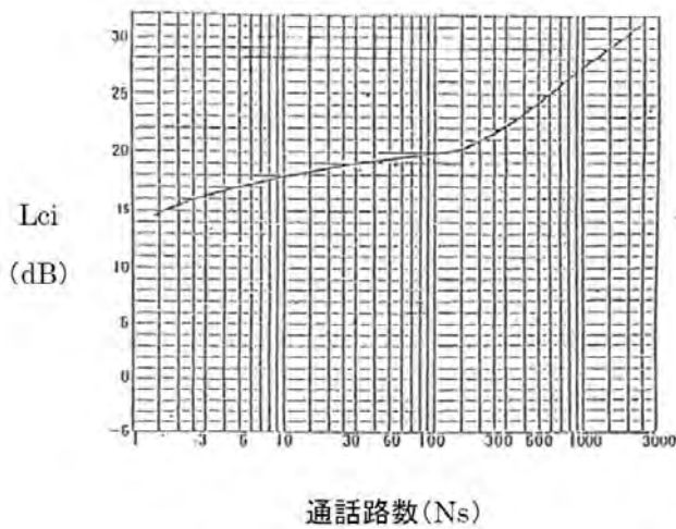
図1 最大負荷係数(Lci)
