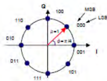
図9 8PSK ビットマッピング
