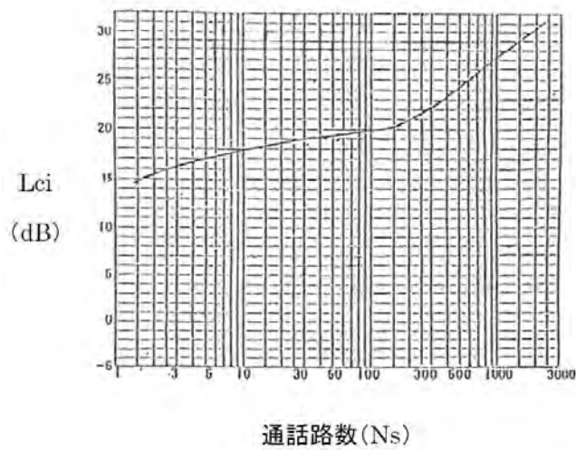
図3-1 最大負荷係数(Lci)
