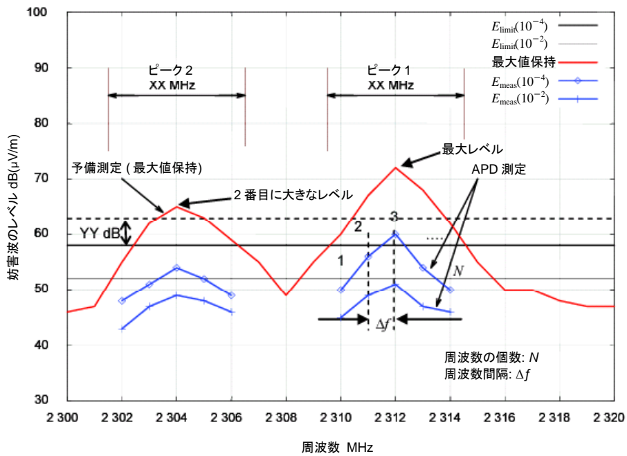
図 C. 1 変動する妨害波の APD 測定 (方法 1) の例
