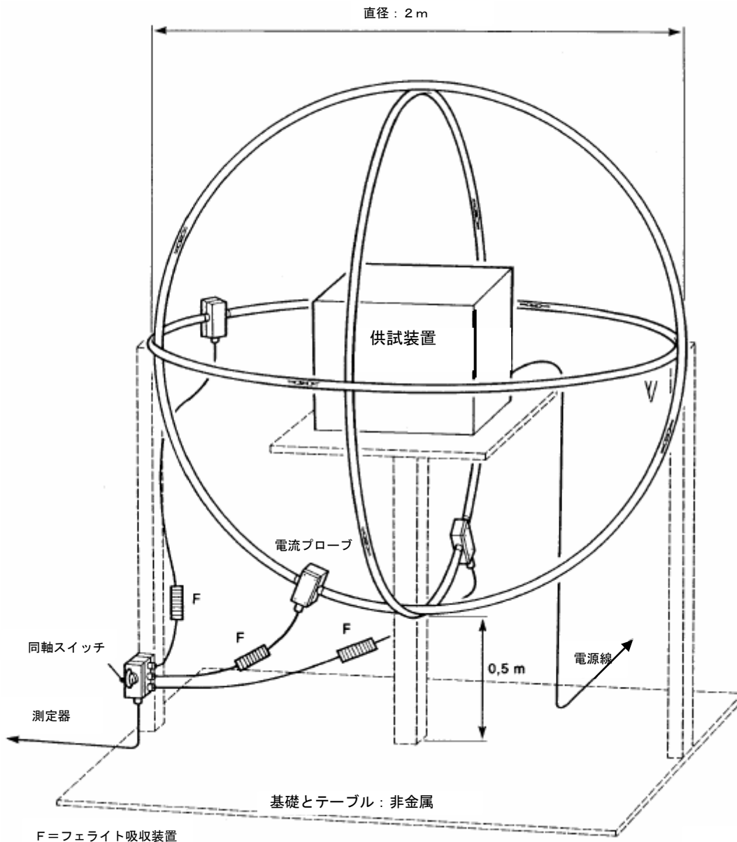
図 18 ループアンテナシステムを使用して行われる磁界誘導電流測定のご概念
