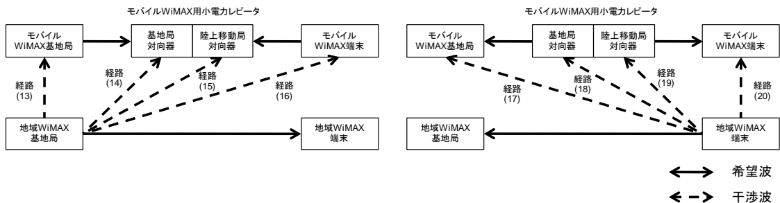
図 2. 4-9 地域 WiMAX からの被干渉経路
