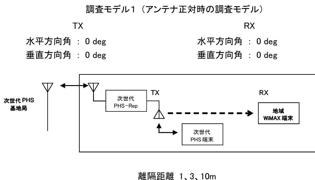
図. 添5-2. 1-1 調査モデル1及び調査モデル1'
