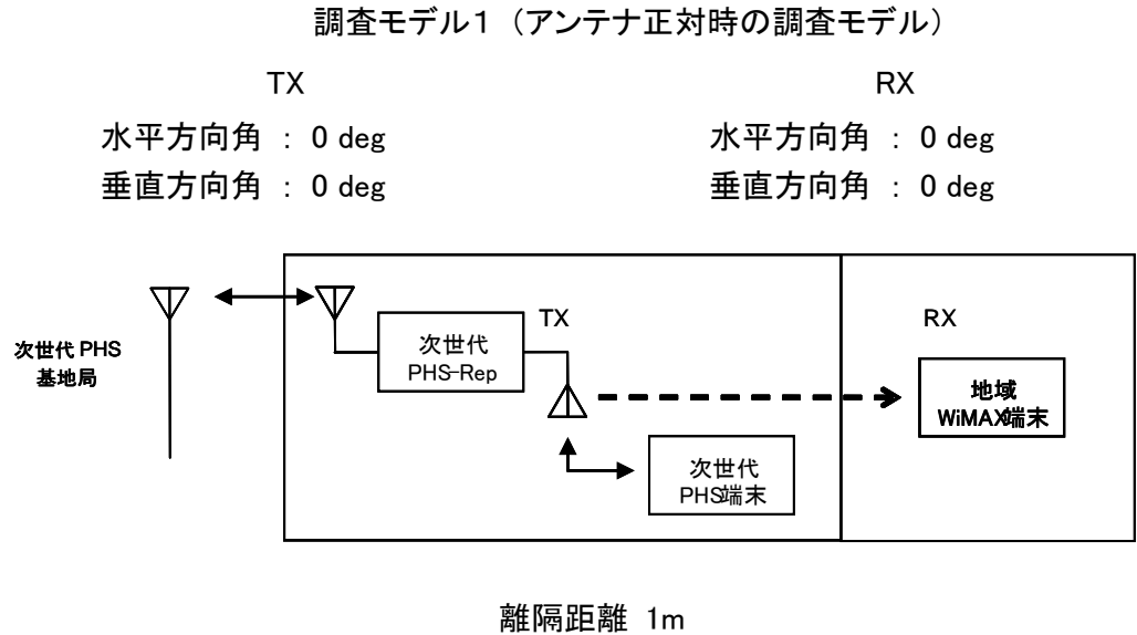
図. 添5-2. 1-6 調査モデル1
