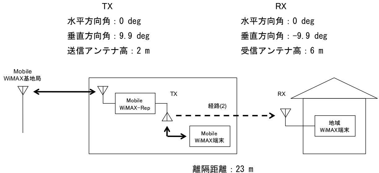
図. 添5-1. 1-6 FWAモデル2（調査モデル2）
