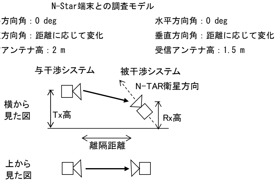
図. 添5-1. 1-16 N-Star端末との調査モデル(垂直)
