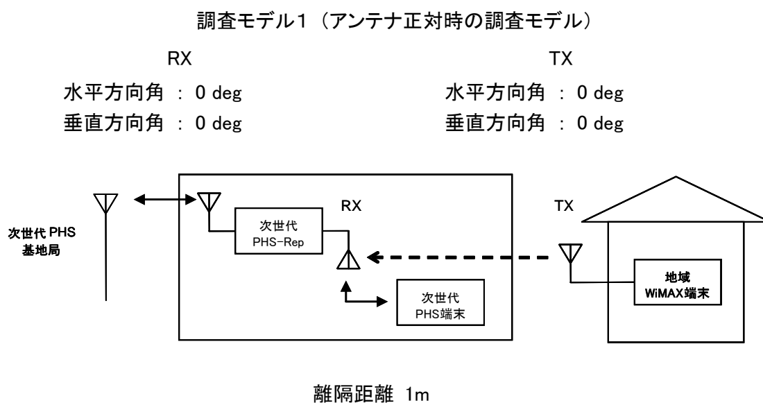
図. 添5-2. 2-8 調査モデル1
