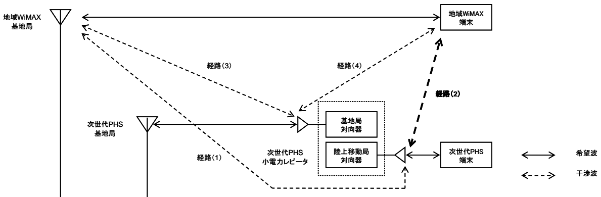
図 2. 5 - 1 次世代 PHS ~地域 WiMAX 間の干渉経路
