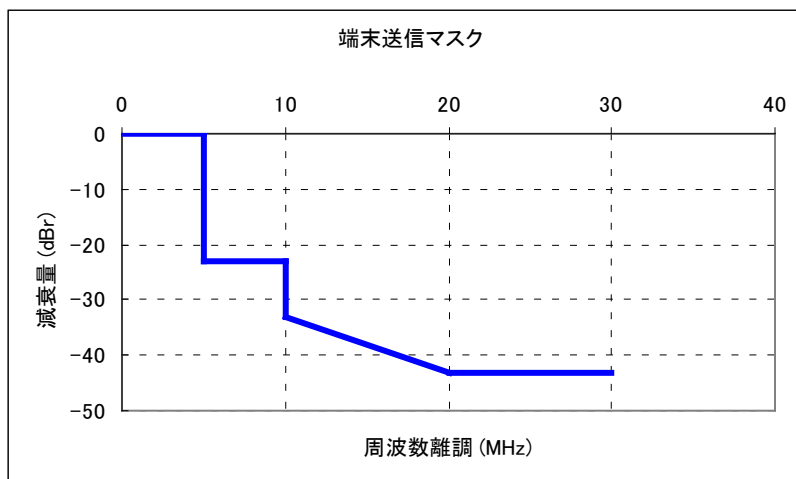
図3 次世代 PHS 端末の送信マスク
