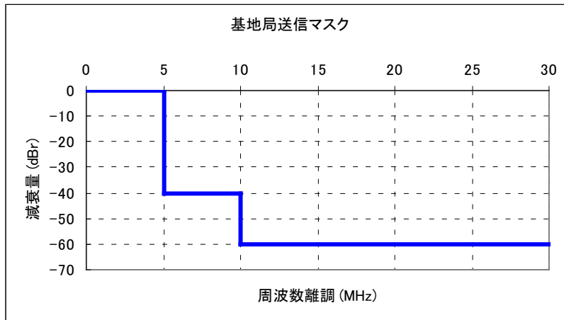
図2 次世代 PHS 基地局の送信マスク
