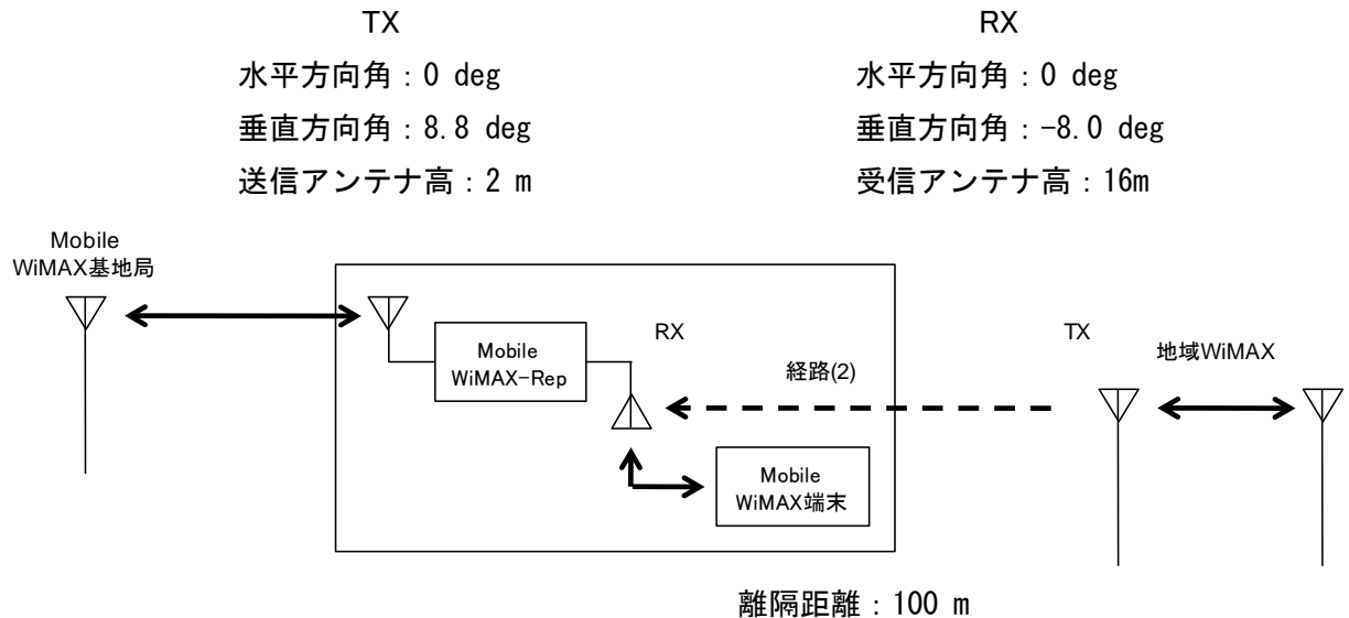
図. 添5-1. 2-7 FWAモデル3（調査モデル2）
