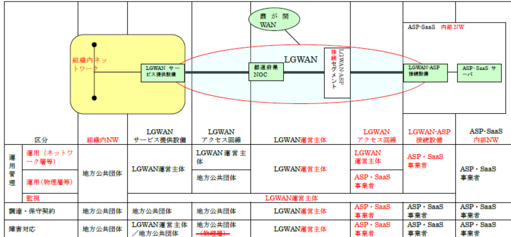
図 4-1 LGWAN-ASPの構成と責任分界
