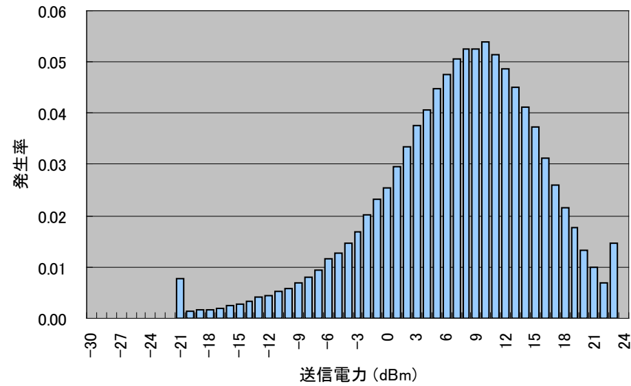
LTE移動局の送信電力分布(LTEチャネル幅20MHz運用例)
