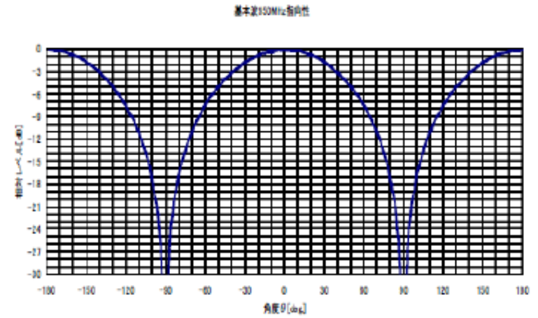
中出力型及び低出力型950MHz帯パッシブタグシステムのリーダ/ライタ並びにアクティブタグシステムのアンテナ指向特性(水平面)
