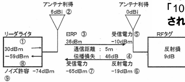
5mシステムの伝播特性(平成17年報告書から引用)
