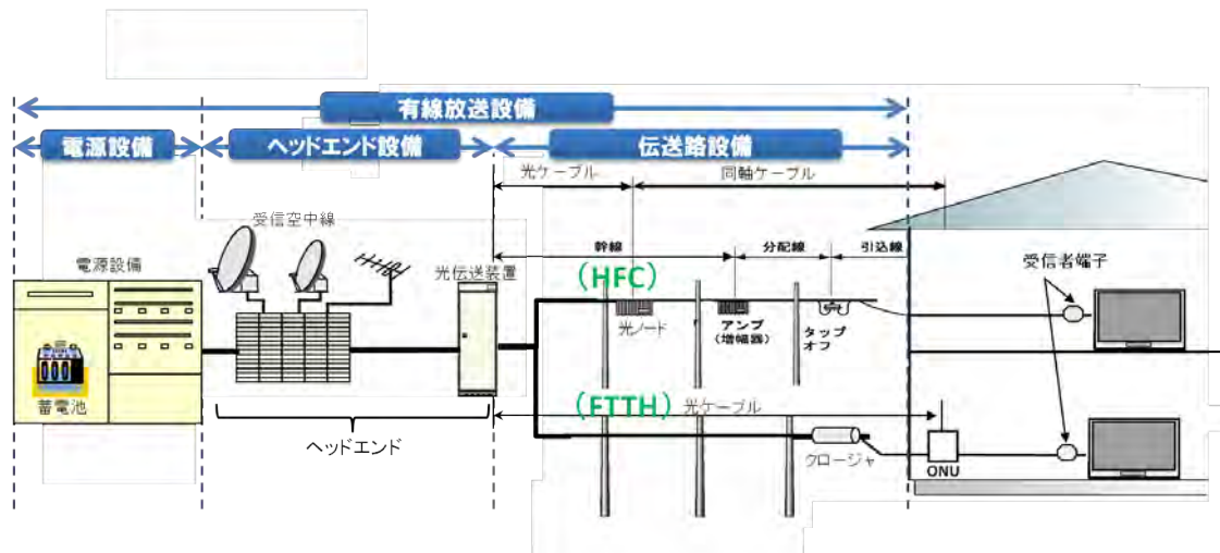
図 2 - 2 有線放送設備構成図 (例)
