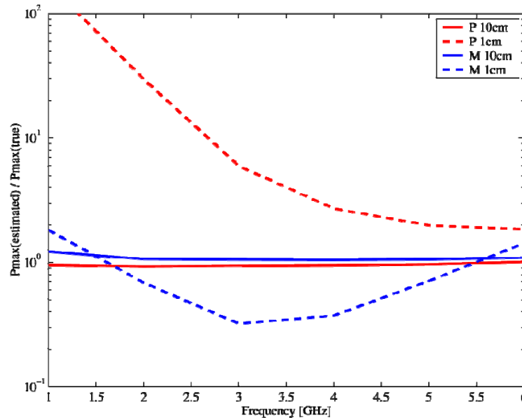
図15 自由空間での電界強度と平面波反射率から推定した人体に入り込む電力密度の対真値比
