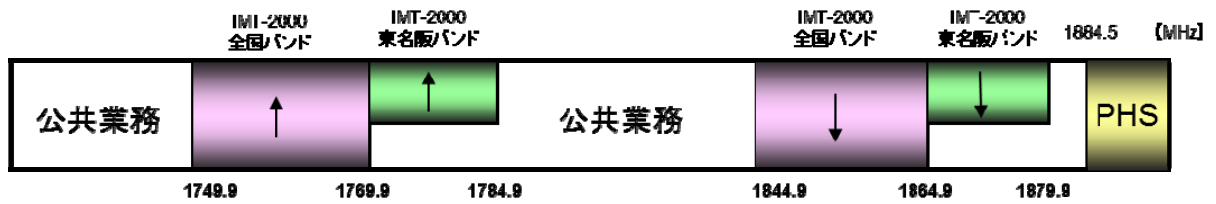
図-四-5-15 1.7GHz 帯携帯無線通信の周波数配置
