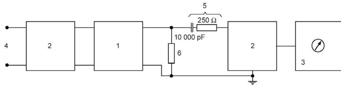
図5 制御装置の測定配置図(5.2.4項参照)
