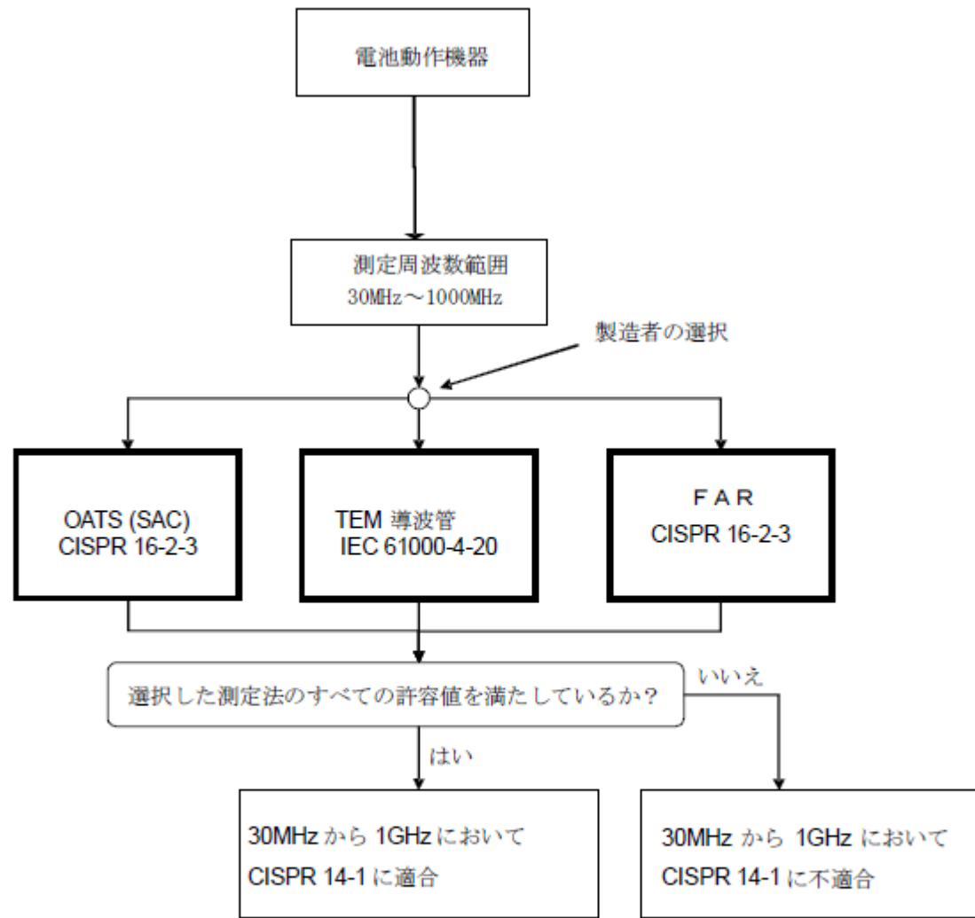
図 11 周波数範囲 30MHz から 1000MHz までの電池動作機器のエミッション試験のフローチャート
