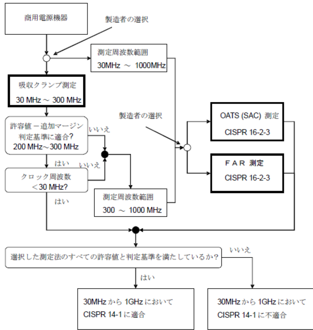
図 10 周波数範囲 30MHz から 1000MHz までの商用電源機器のエミッション試験のフローチャート
