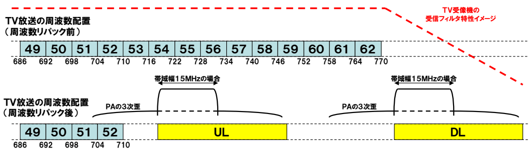
図2. 4. 3. 2-1 追加検討で想定する周波数配置
