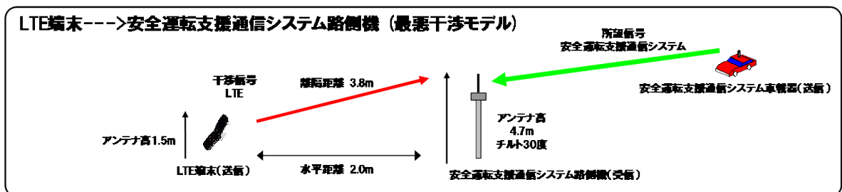
図 2. 5. 3-3 LTE移動局からITS路側機への与干渉モデル
