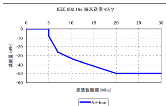
図. 参 1-3-6 地域 WiMAX 移動局の送信マスク (10MHz システム)
