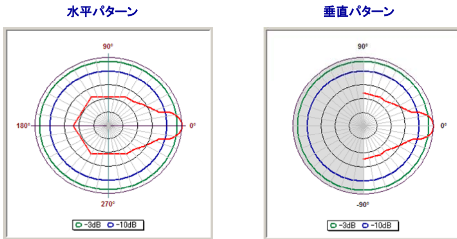
図. 参1-3-10 高利得 FWA の移動局 (モデル2) のアンテナパターン
