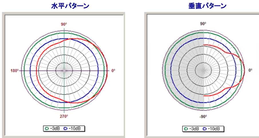
図. 参1-3-9 高利得 FWA の移動局 (モデル1) のアンテナパターン
