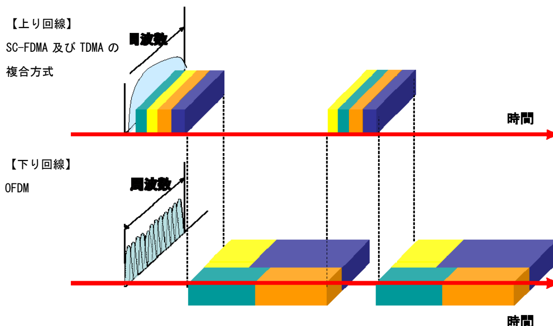
図 1. 5. 1-1 SC-FDMA 及び TDMA の複合方式のイメージ
