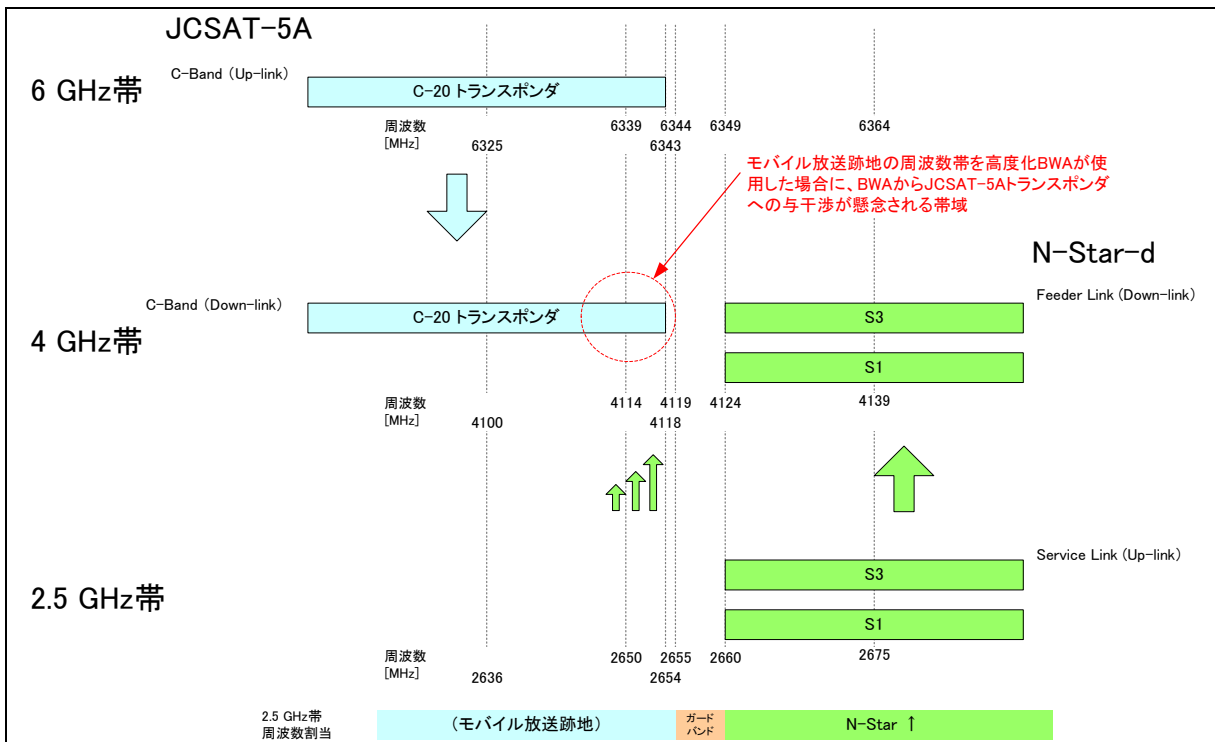
図. 参 1 - 4 - 5 N-Star 衛星・JCSAT-5A トランスポンダの周波数配列
