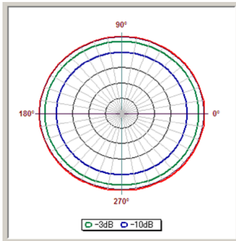
図. 参1-3-7 高利得FWAの基地局(モデル1, 2)のアンテナパターン
