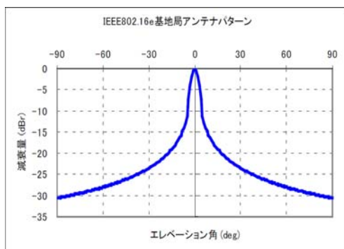
図. 参 1-3-3 地域 WiMAX 基地局のアンテナパターン
