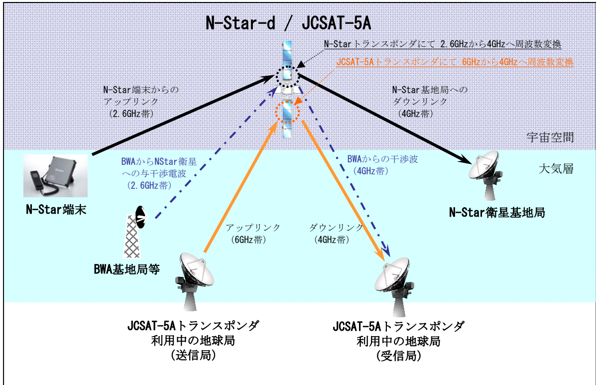
図. 参 1 - 4 - 4 N-Star・JCSAT-5A・BWA 干渉イメージ図
