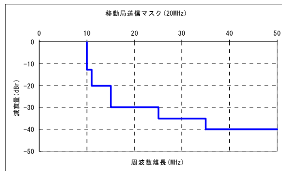
図. 参 1-1-4 XGP 移動局および小電力レピータ送信マスク (20MHz システム)
