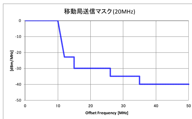
図. 参 1-2-3 モバイル WiMAX 移動局の送信マスク (20MHz システム)
