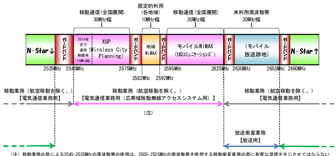
図4. 1. 1-1 周波数の分配と割当状況
