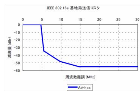
図. 参 1-3-1 地域 WiMAX 基地局の送信マスク (10MHz システム)
