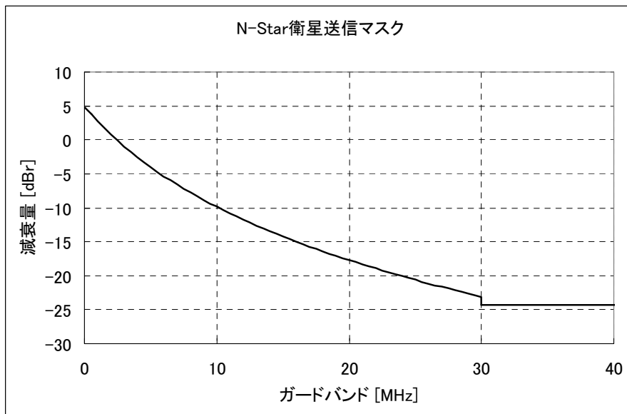
図. 参 1 - 4 - 3 N-Star 衛星の送信マスク
