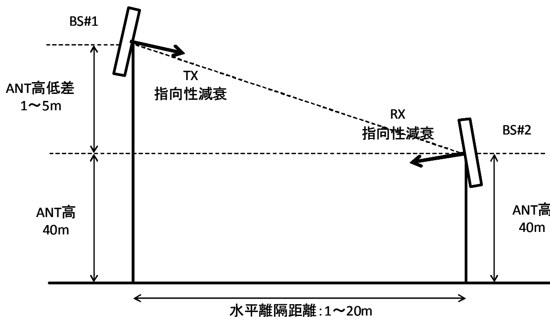
図. 参3-参考1 サイトエンジニアリングによる干渉検討イメージ
