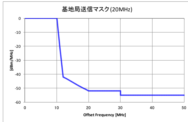
図. 参 1-2-1 モバイル WiMAX 基地局の送信マスク (20MHz システム)
