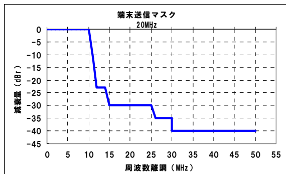
図. 参 1-3-5 地域 WiMAX 移動局の送信マスク (20MHz システム)
