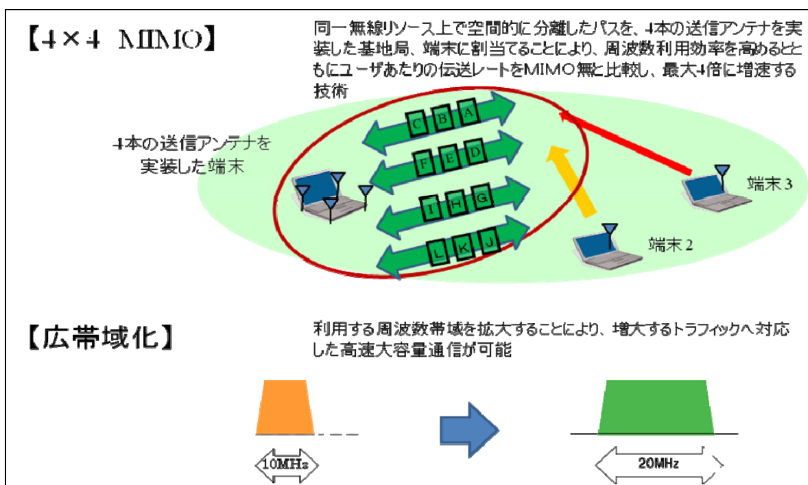
図 3. 2. 2-1 モバイル WiMAX の技術的条件について
