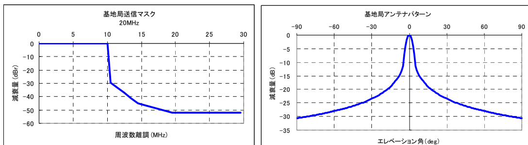
図. 参 1-1-2 XGP 基地局送信マスク (20MHz システム) および XGP 基地局アンテナパターン
