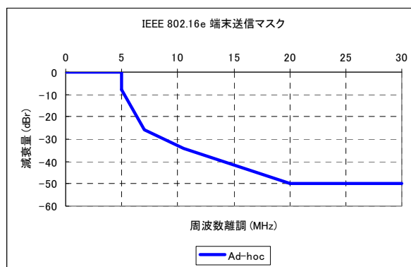
図. 参 1 - 3 - 1 3 高利得 FWA の移動局の送信マスク (10MHz システム)
