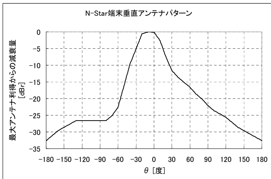
図. 参 1-4-1 N-Star 端末のアンテナパターン (垂直方向)
