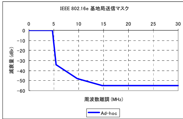
図. 参 1 - 3 - 1 2 高利得 FWA の基地局の送信マスク (10MHz システム)
