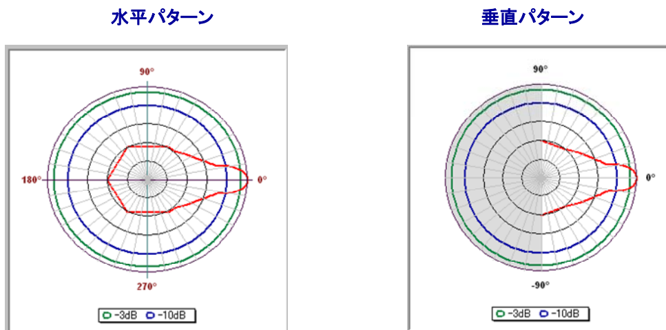
図. 参1-3-11 高利得 FWA の移動局 (モデル3) のアンテナパターン
