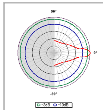
図. 参1-3-8 高利得FWAの基地局(モデル3)のアンテナパターン
