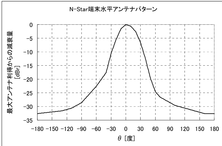
図. 参 1 - 4 - 2 N-Star 端末のアンテナパターン (水平方向)
