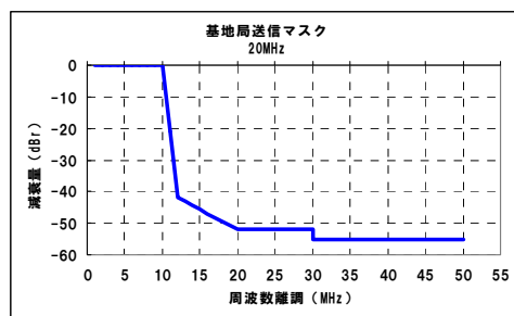
図. 参 1-3-2 地域 WiMAX 基地局の送信マスク (20MHz システム)
