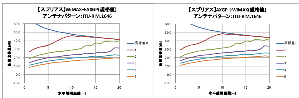
図. 参3-参項2 サイトエンジニアリングを考慮した所要改善量の一例(スプリアス)
