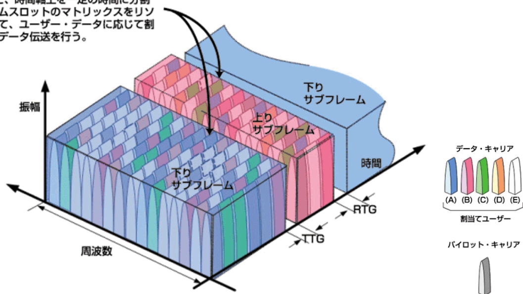
図 1. 5. 2 - 1 モバイル WiMAX (OFDMA/TDD 方式) のデータ割当てイメージ
