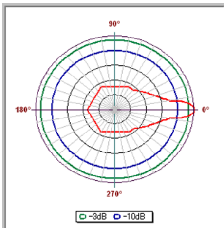
図. 参1-3-8 高利得FWAの基地局(モデル3)のアンテナパターン
