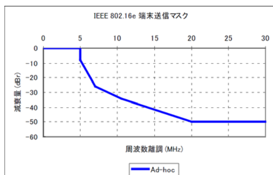
図. 参 1-3-4 地域 WiMAX 移動局の送信マスク (10MHz システム)
