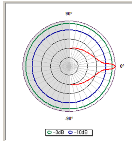
図. 参1-3-7 高利得FWAの基地局(モデル1, 2)のアンテナパターン
