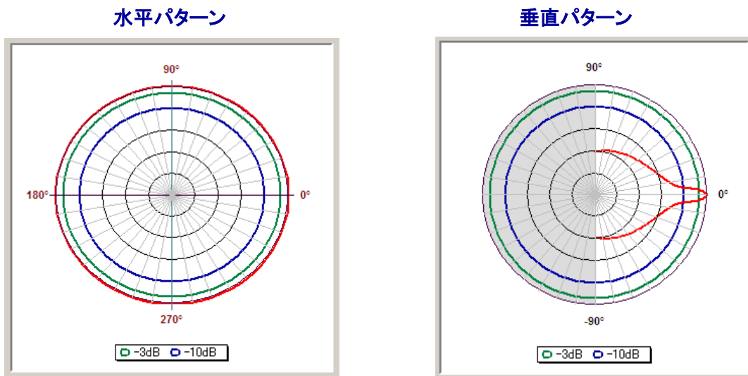
図. 参1-3-7 高利得FWAの基地局(モデル1, 2)のアンテナパターン
