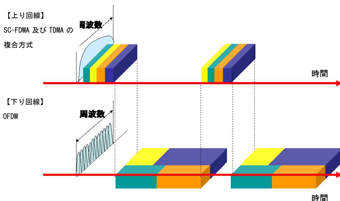
図 1. 5. 1-1 SC-FDMA 及び TDMA の複合方式のイメージ
