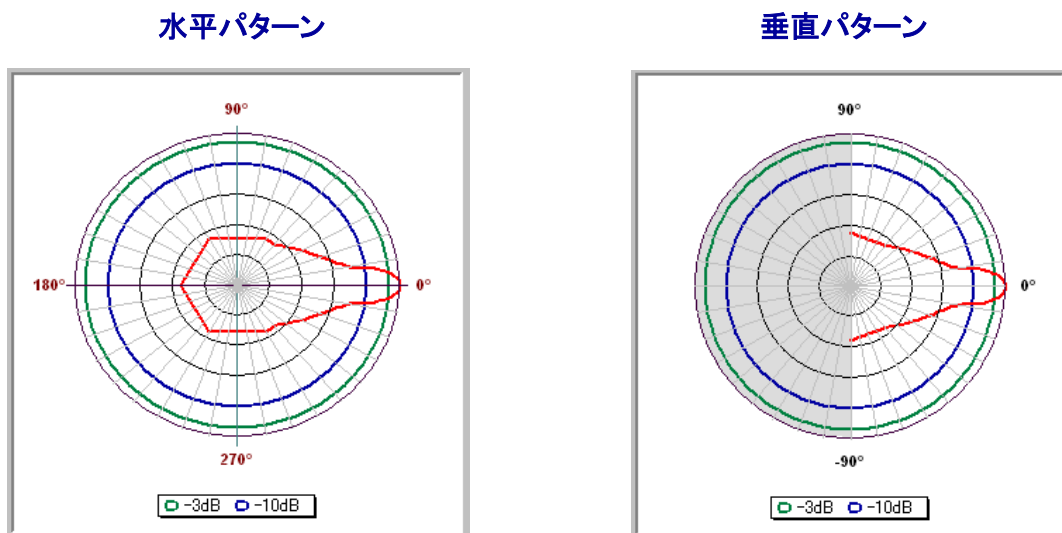
図. 参1-3-8 高利得FWAの基地局(モデル3)のアンテナパターン
