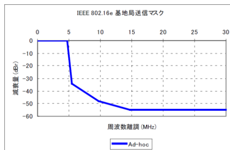
図. 参 1-3-1 地域 WiMAX 基地局の送信マスク (10MHz システム)
