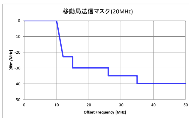
図. 参 1-2-3 モバイル WiMAX 移動局の送信マスク (20MHz システム)
