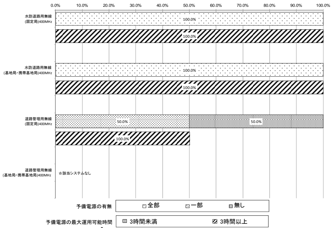
図表－５－６－１５ 予備電源保有状況及び予備電源の最大運用可能時間 (水防道路用無線・道路管理用無線)(内訳)【北陸】
