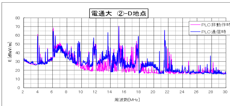
図4.9 電気通信大学多摩川グラウンド管理棟での電界測定結果例
