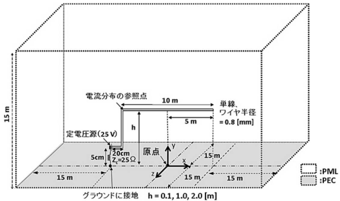
図2.1 解析モデル
