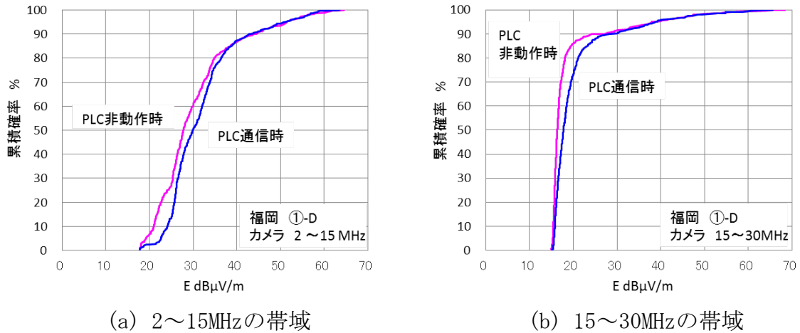
図4.21 福岡HD-PLC検証ハウス（カメラ I）での累積確率分布特性(①-D地点)
