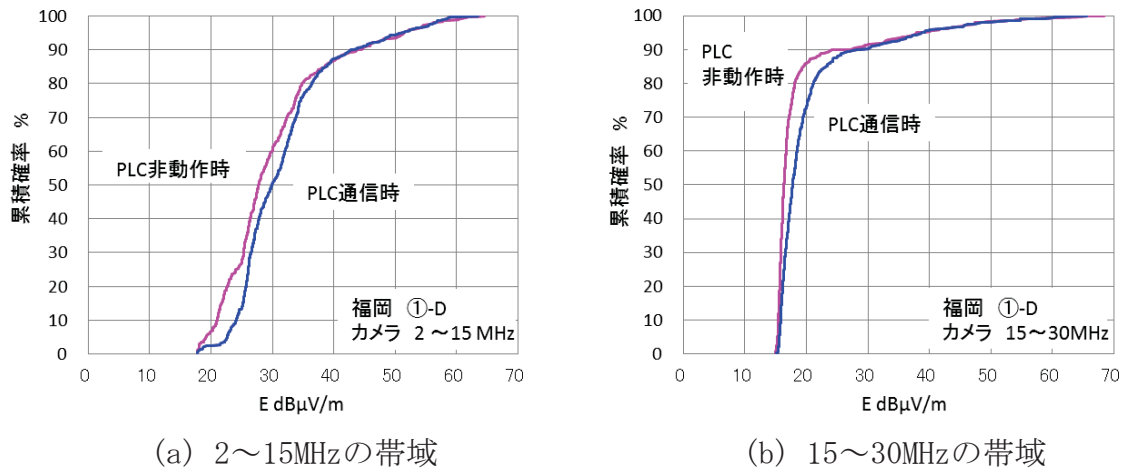
図4.21 福岡HD-PLC検証ハウス（カメラ I）での累積確率分布特性(①-D地点)
