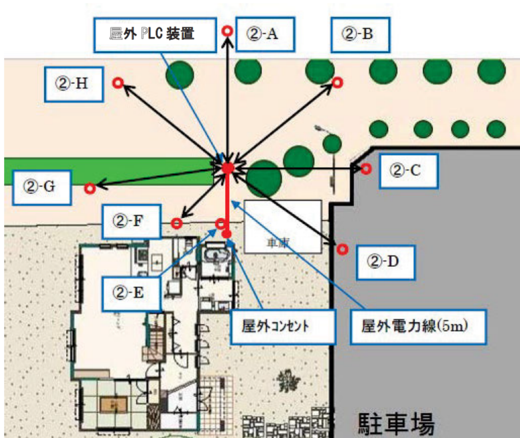
図4.22 福岡HD-PLC検証ハウス(カメラII)
