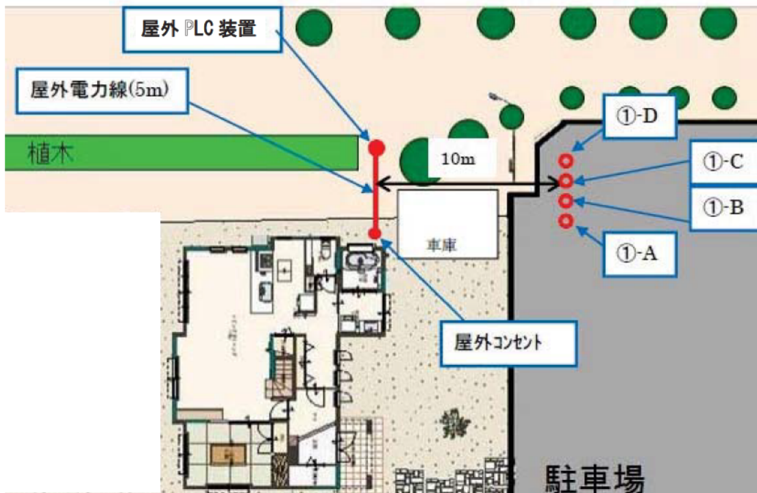
図4.13 福岡HD-PLC検証ハウス(カメラ I)
