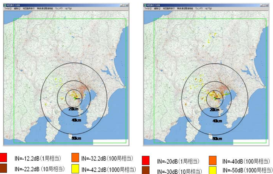
図 2. 5. 2-6 複数の基地局からの干渉影響（通常の基地局） （許容干渉レベルとして、左図は I/N = -12.2 dB、右図は I/N = -20 dB）
