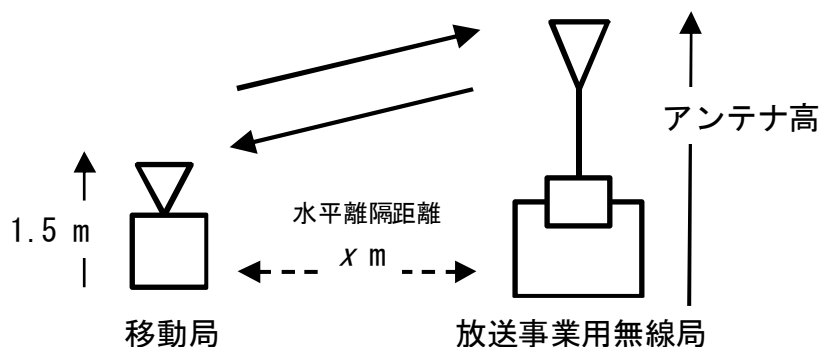
図 2. 4. 3-1 移動局との干渉検討モデル
