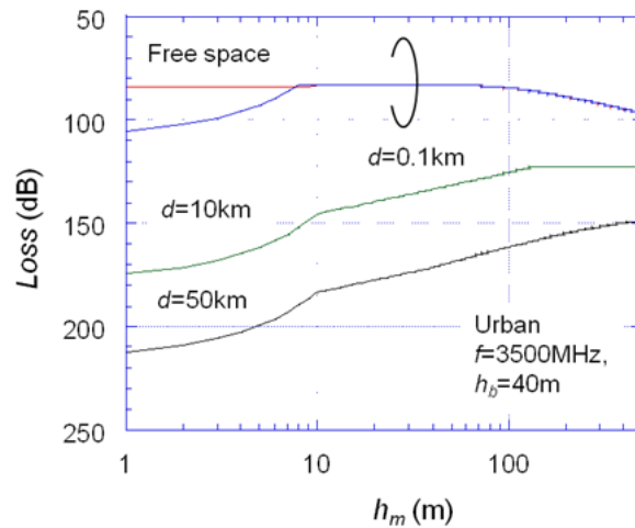
図 1.2-4 移動局高特性
