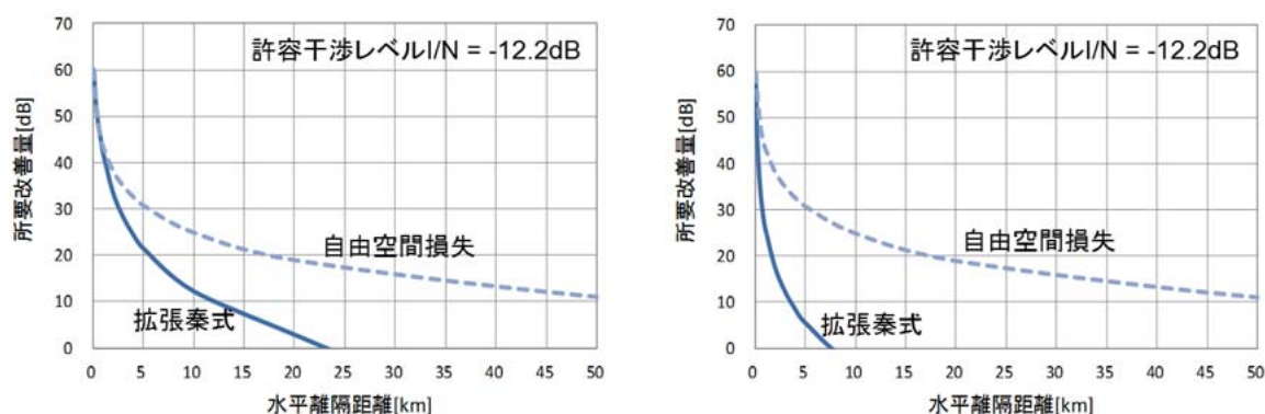
図 2. 5. 2－4 用いる伝搬式の影響 (同一チャネル干渉、小セル基地局のアンテナ高が左図は 10 m、右図は 5 m)
