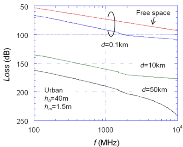
図 1.2-2 周波数特性
