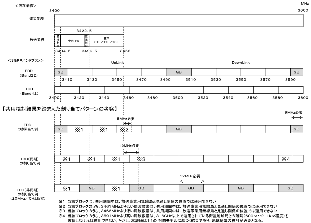
図2. 7. 4-1 3.4~3.6GHz帯において想定される割り当てパターン例
