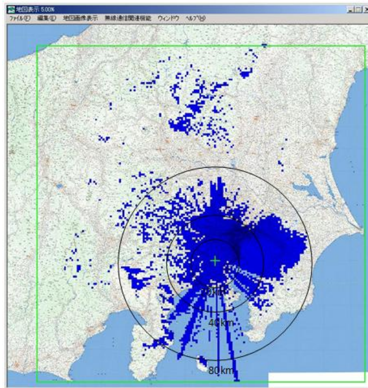
(d) 許容干渉レベル I/N = -42.2\text{dB} (基地局 1,000 局以下で許容干渉レベルを超過) 図 2. 5. 3-5 複数の通常基地局からの同一チャネル干渉の影響の一例 (地球局 A)
