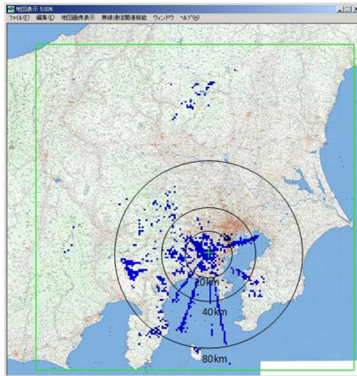
図 2. 5. 3-6 複数の小セル基地局からの同一チャネル干渉の影響の一例 (サイトシールディングあり) (地球局 A)
