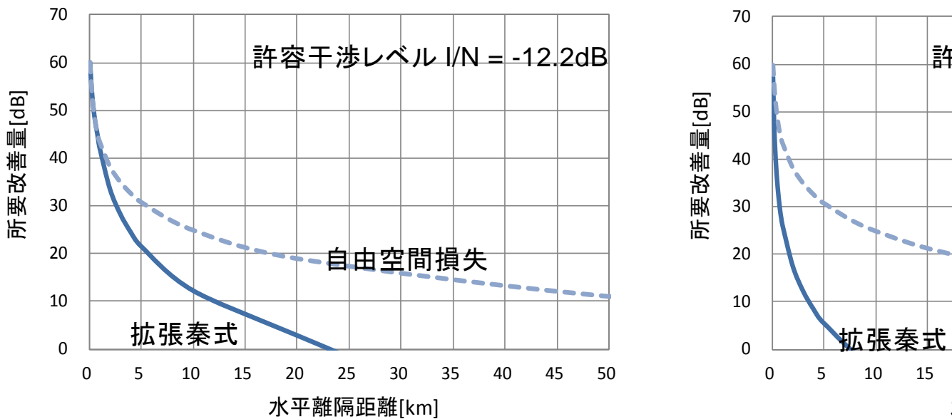
図 2. 5. 3-4 用いる伝搬式の影響
