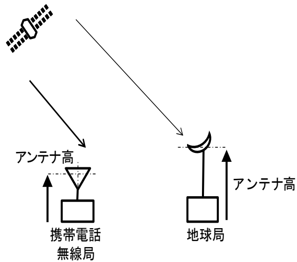
図 2.5.2-2 人工衛星局との干渉検討モデル
