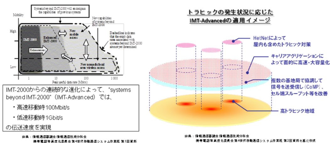
図1. 4-1 第4世代移動通信システムの基本コンセプト
