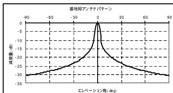
図. 参1-1-2 基地局送信マスク (10/20MHz システム) 及び基地局アンテナパターン
