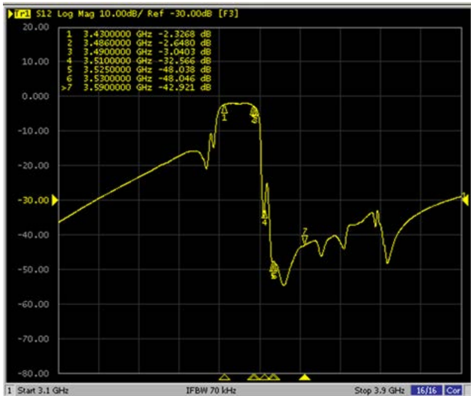
図 参 7.3.2-5 DUP2 の通過特性 (Tx→ANT)
