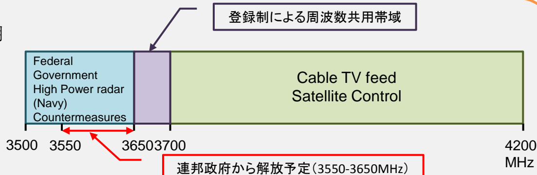
米国における3.5 - 4.2GHz帯の割当て状況
