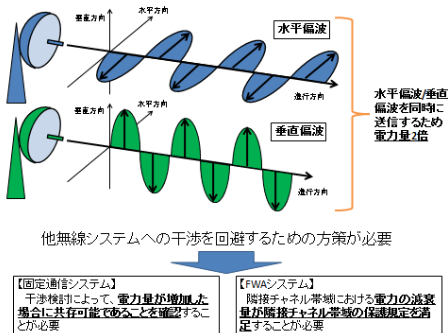
図 2-6 コチャネル配置時における干渉回避の方策
