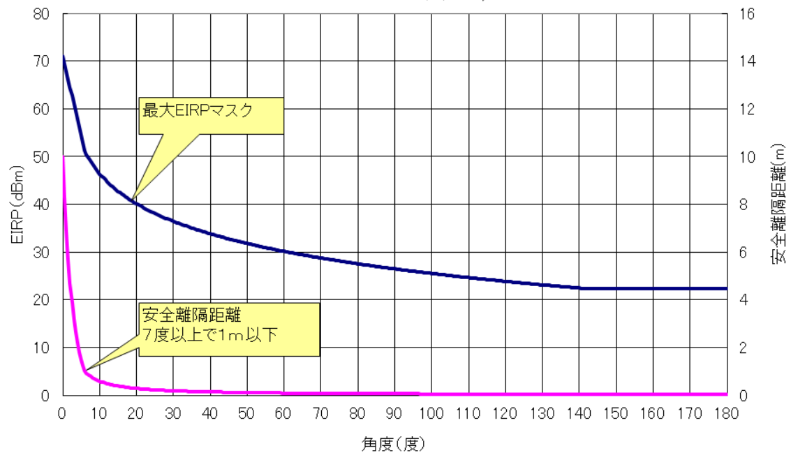
最大EIRP規格と安全離隔距離 38GHz帯(FWA)
