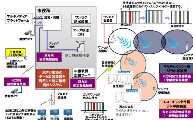
図5 耐災害性の強い放送系技術を用いた防災システムの研究開発
