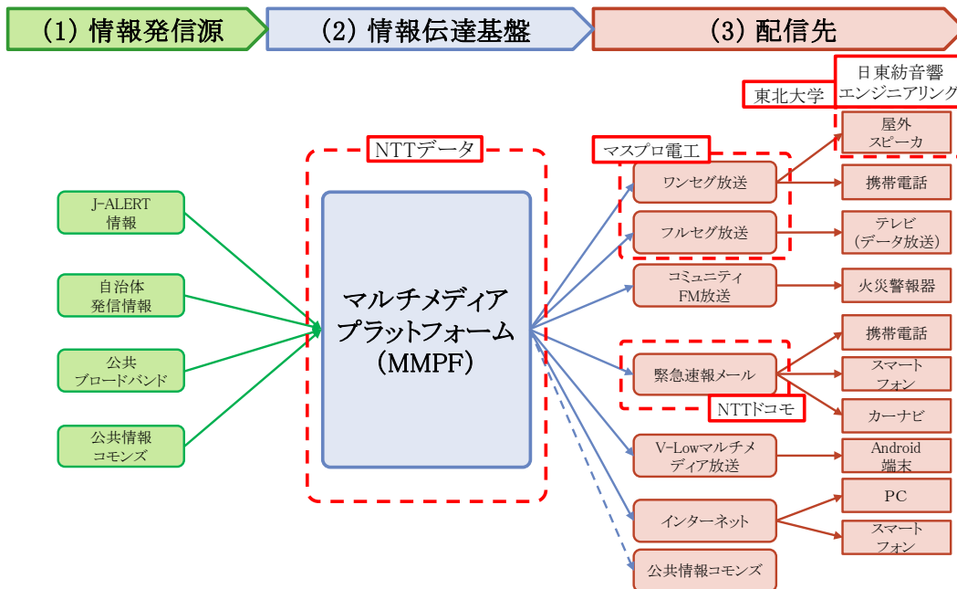
図3 災害情報伝達システムのモデルおよび研究開発範囲
