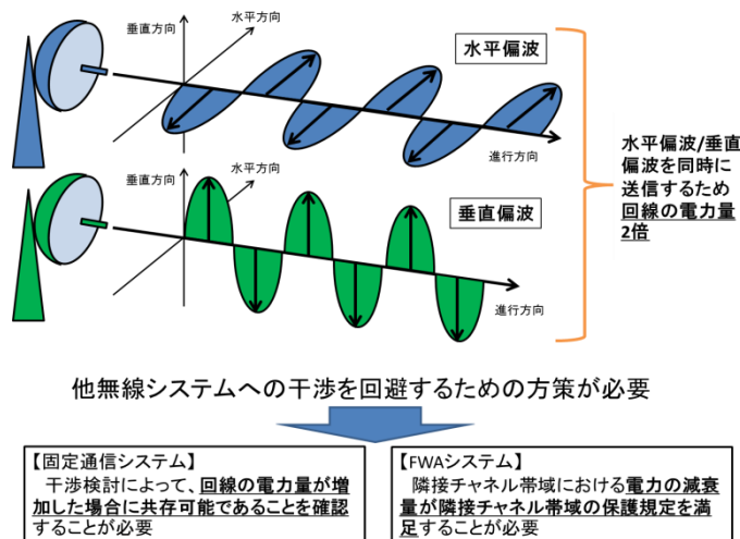
図9 交差偏波多重方式の導入時における干渉回避方策
