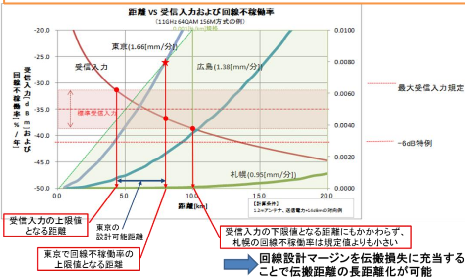
図12 伝搬距離と受信入力/回線不稼働率の地域による違い
