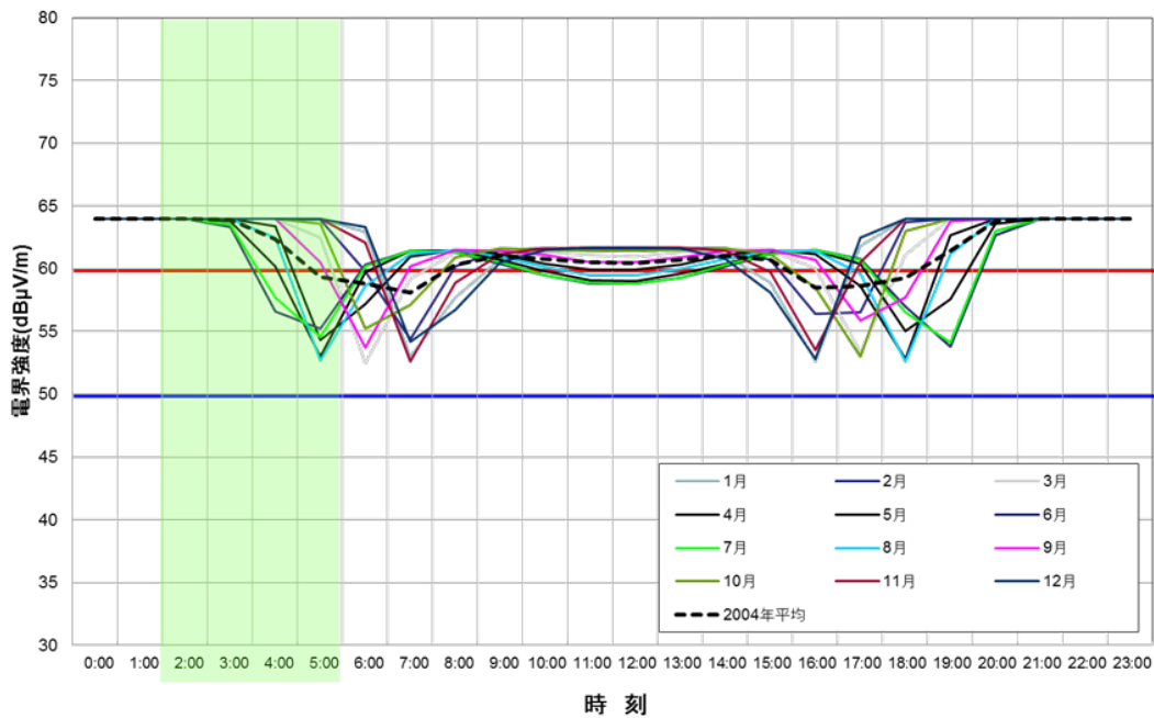
図 3.2-6 各時刻における電界強度のシミュレーション値（2004年月平均値） 送信所：おおたかどや山（40kHz） 受信場所：稚内市
