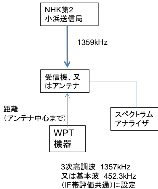
図 3. 7. 2-6 (b) アンテナ、受信機、WPT システム等の位置関係
