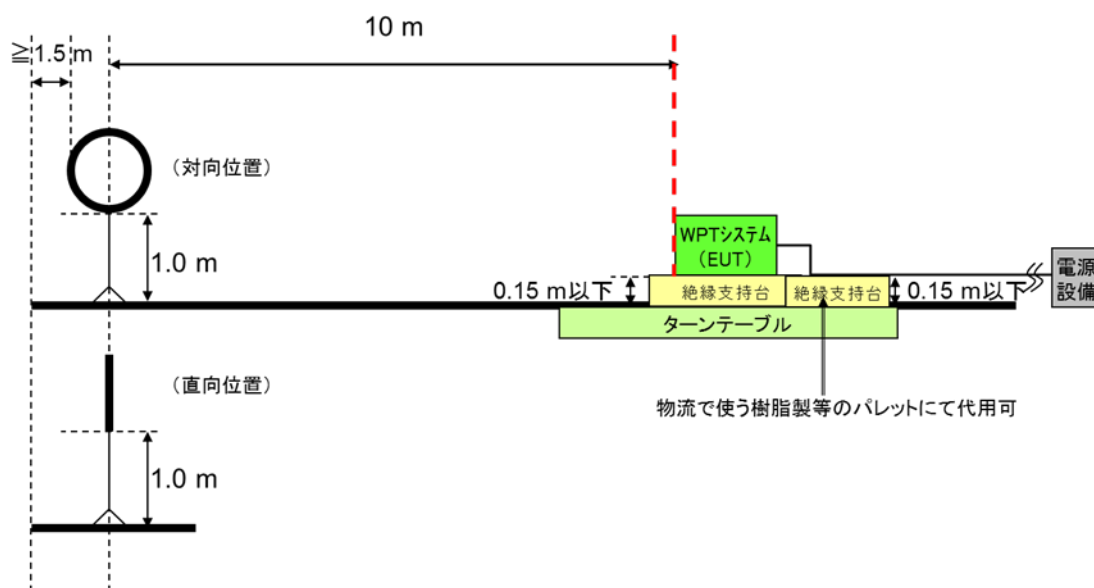
図 C.3-2 電気自動車用 WPT システムの放射妨害波測定 (9 kHz～30 MHz)
