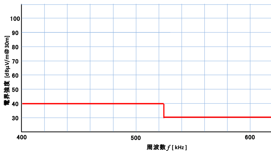
図 3.1-11 目標値として設定した家電機器用 WPT システム③の漏えい電界強度 II
