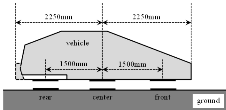
302 図 G. 2. 5. 1-1 車両モデルの概観と伝送システム搭載位置
