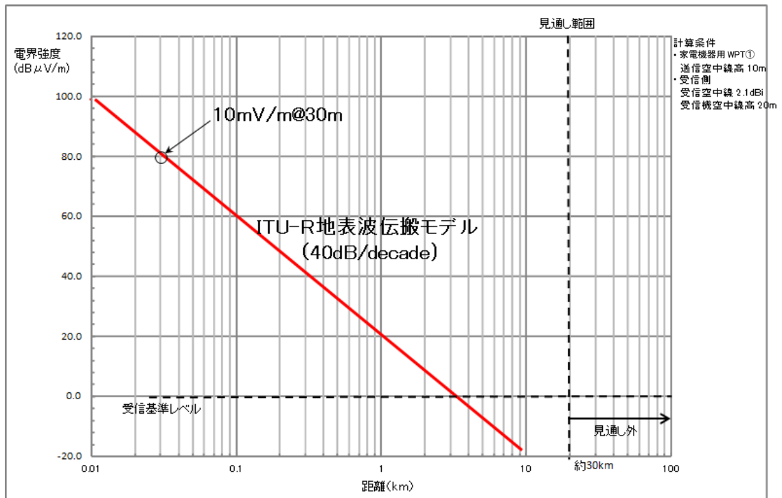
図 3.8.3 家電機器用 WPT システム①の漏えい電界の伝搬特性計算値
