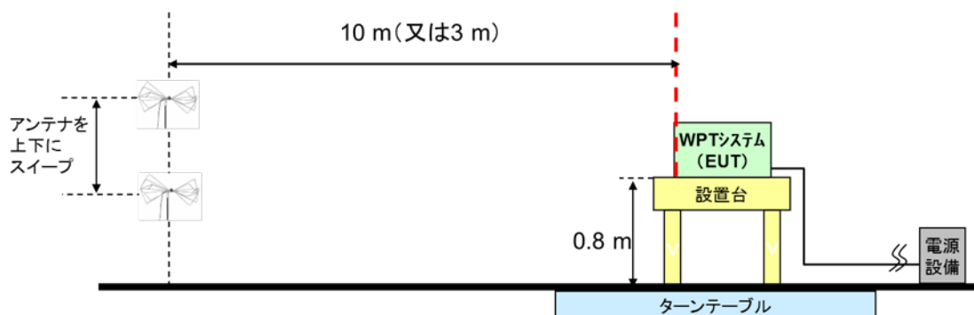
図 C.3-5 家電機器用 WPT システムの放射妨害波測定 (30 MHz～1 GHz)
