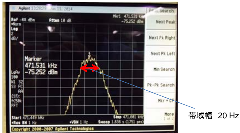
図 3.3.3-6 基本波の周波数スペクトラム
