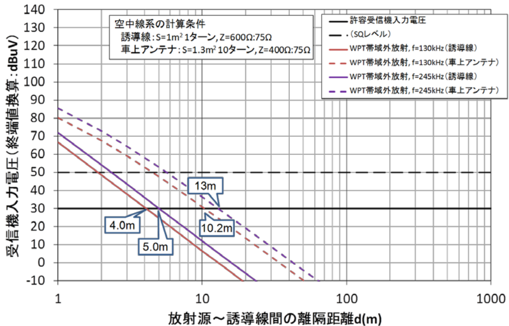
図3. 4. 2-7 所要離隔距離の計算結果 (家電機器用WPTシステム②・帯域外放射)
