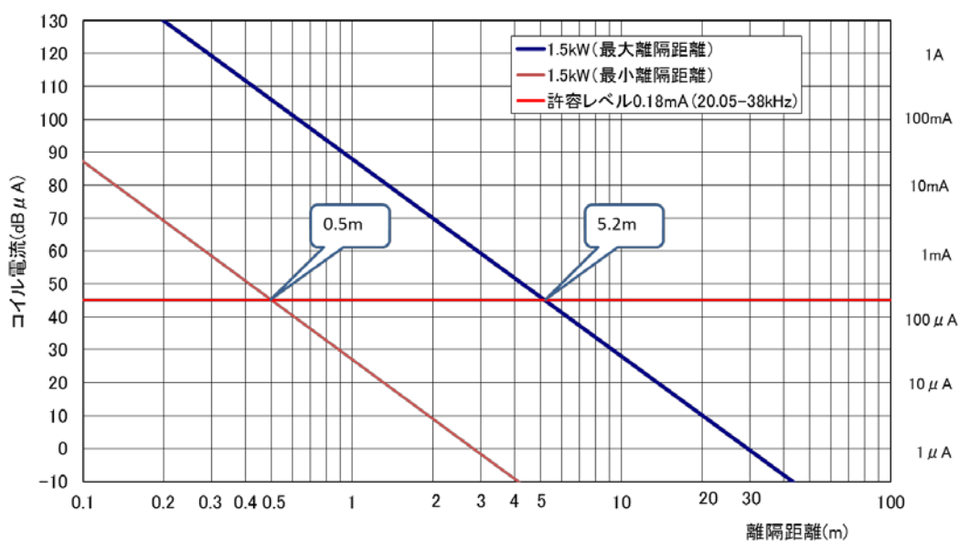
図 3.3.2-5 信号保安設備「Type B」装置の許容電流値（実効値）と所要離隔距離
