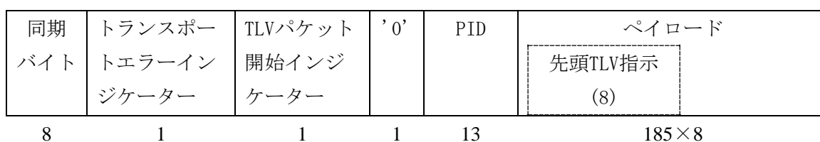
図 6.6-2 分割 TLV パケットの構成
