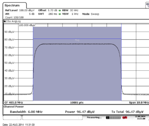
図 2.2-17 J.83C 256QAM U15(485MHz)
