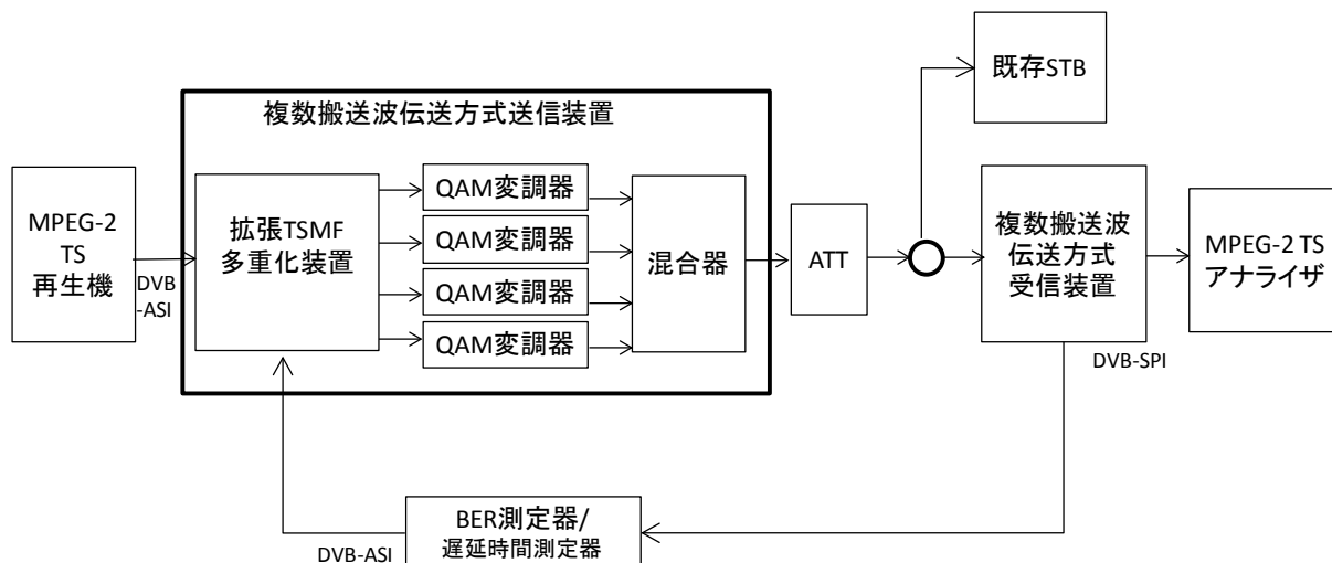
図 1 実験系統
