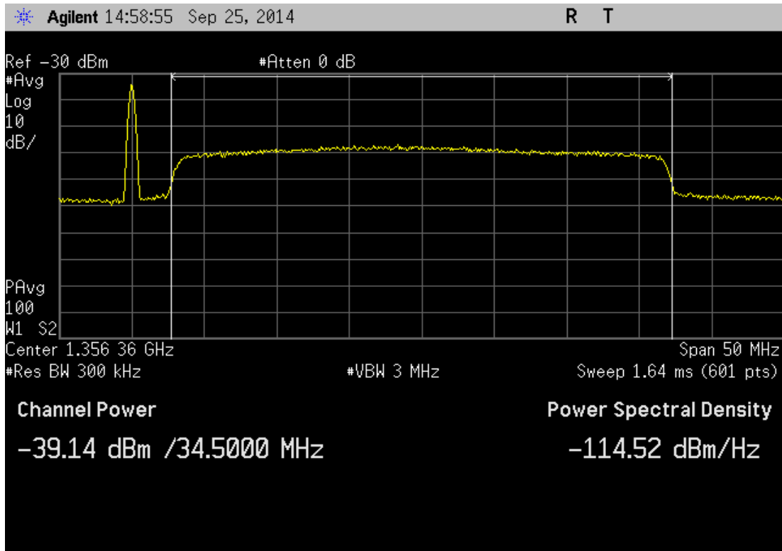
写 2.4-3 16APSK(7/9) 妨害波 f_c - 20\text{MHz} (1336.36MHz)、UD 比 5dB
