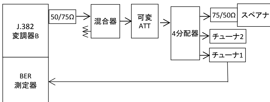
図 2.11-1 J.382 信号のハム変調特性の測定系統図
