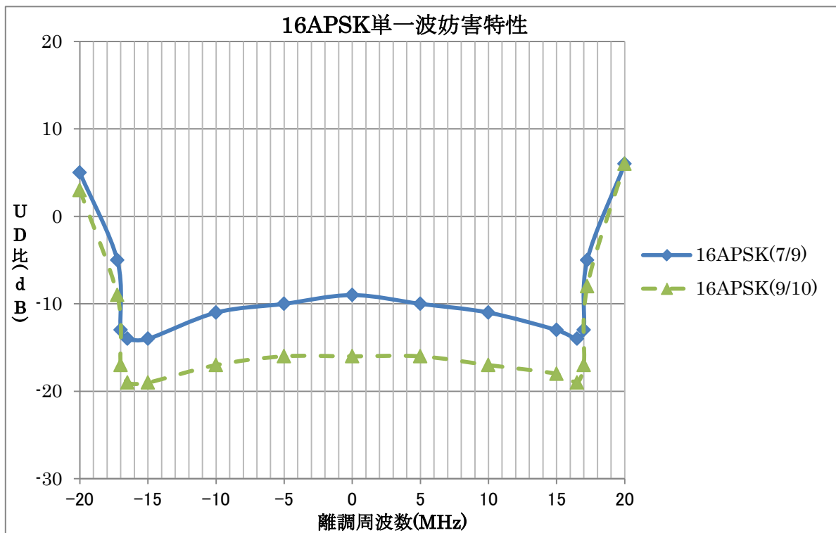
図 2.4-2 16APSK(7/9),(9/10) 信号の単一波信号妨害による UD 比
