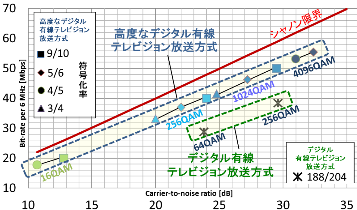
図 7.2-4 高度なデジタル有線テレビジョン放送方式のLDPC符号による符号化利得と所要CN比(理論値)
