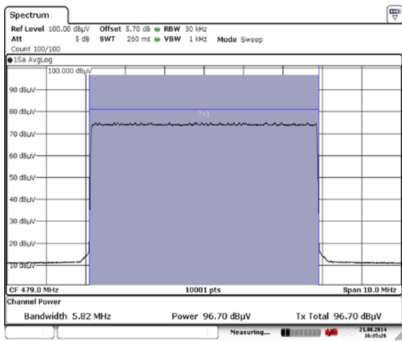
図 2.2-2 J.382 16QAM(4/5) U14(479MHz)
