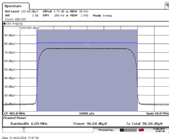
図 2.2-13 J.83C 64QAM U15(485MHz)
