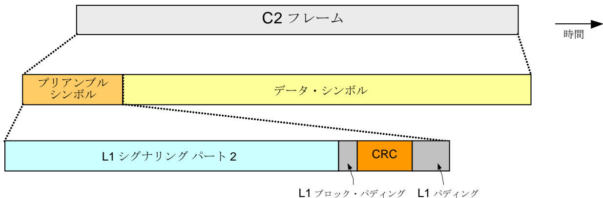
図 7.4-18 L1パート2シグナリングの構成
