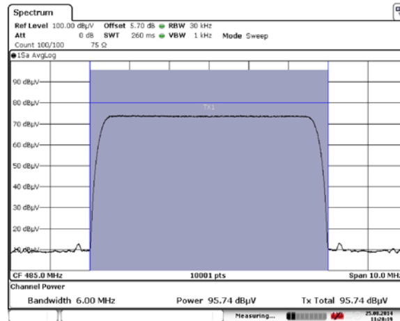
図 2.2-45 J.83C 64QAM U15(485MHz)
