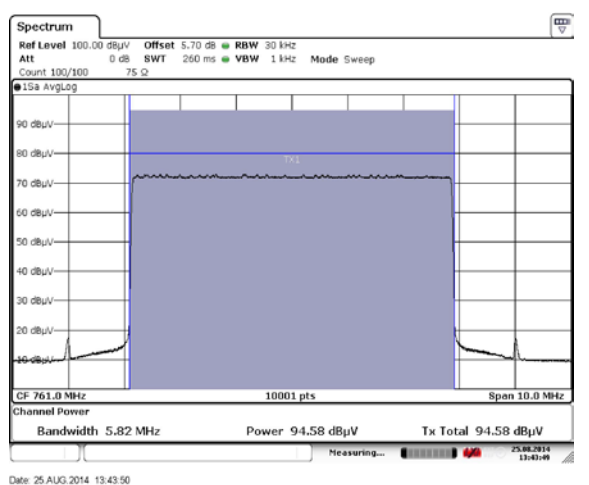
図 2.2-41 J.382 4096QAM(9/10) U61(761MHz)
