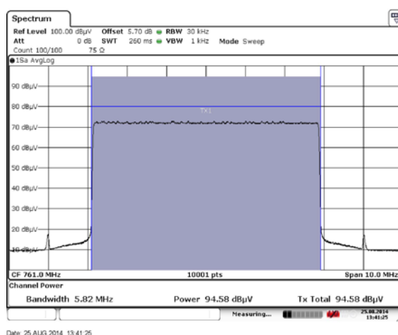
図 2.2-37 J.382 1024QAM(9/10) U61(761MHz)
