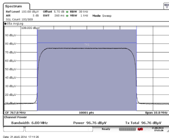
図 2.2-15 J.83C 64QAM U62(767MHz)
