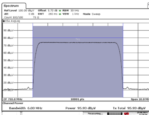
図 2.2-46 J.83C 64QAM U60(755MHz)
