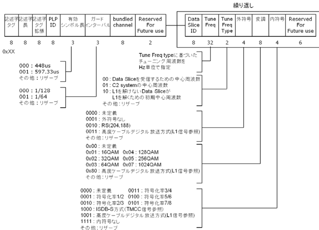
図2.2-2 データ構成
