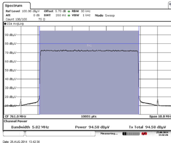
図 2.2-39 J.382 4096QAM(5/6) U61(761MHz)
