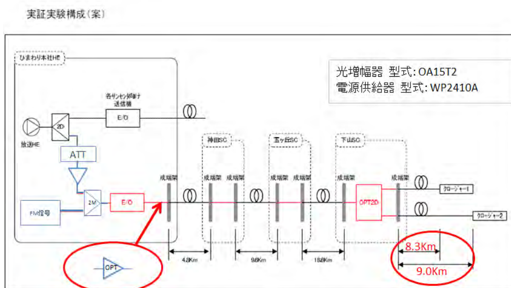
図5 送信点1と送信点2のクロージャーマでの光ケーブル長
