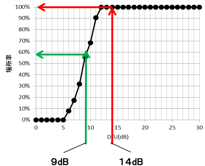
評価3以上が得られるD/U [遅延時間20 \mu s(音楽)]
