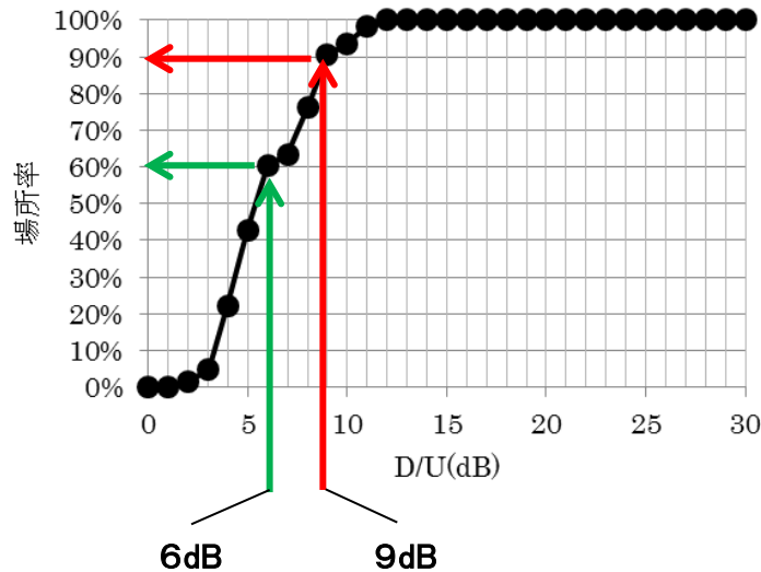
評価3以上が得られるD/U [遅延時間10 \mu s(音楽)]
