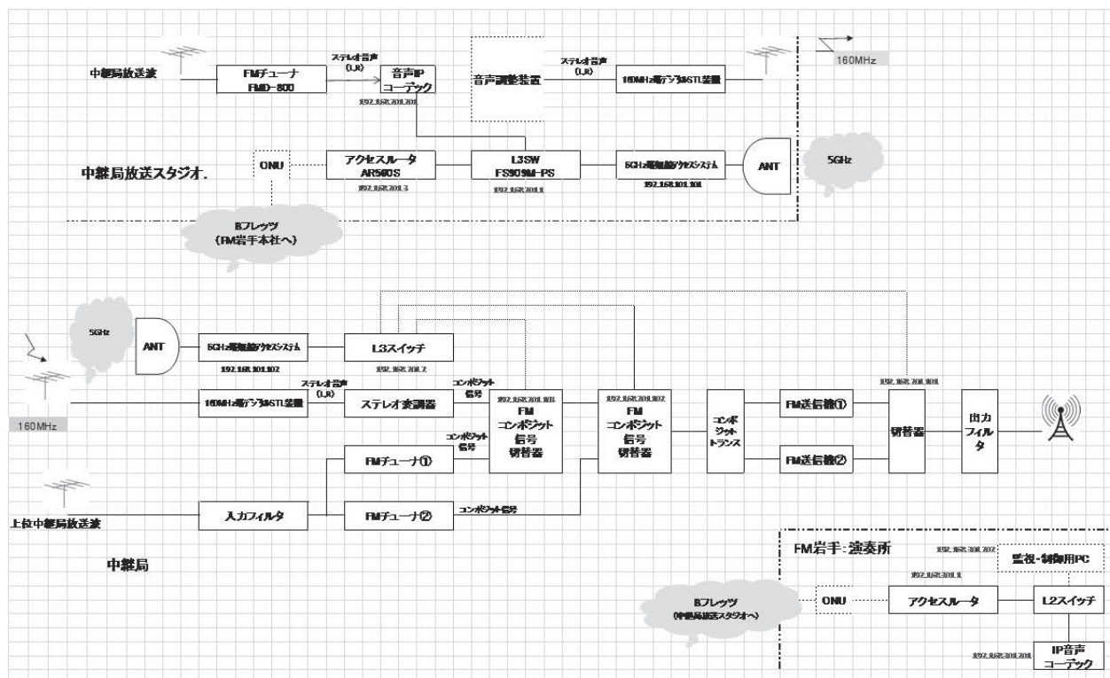
機器構成図
