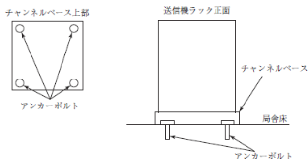
第15図 機器ラックを床に固定する例
