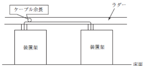
第16図 ケーブルの余長により引っ張りに対応する敷設の例
