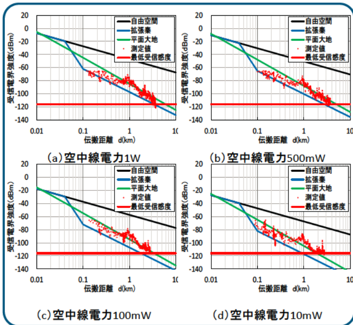
図4-14 受信電力の距離特性結 (熊本合同庁舎 ロングアンテナ)
