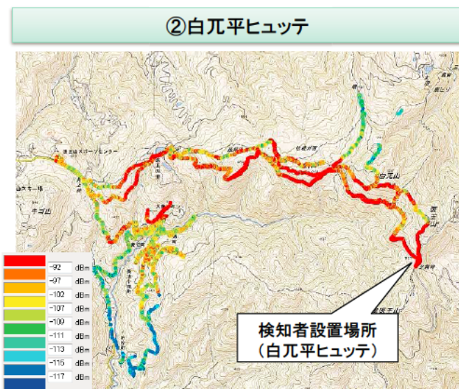
白兀平ヒュッテに設置した検知者端末における登山者端末からの受信電力マップ
