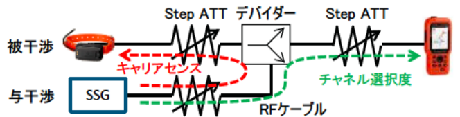
図4-23 測定構成
