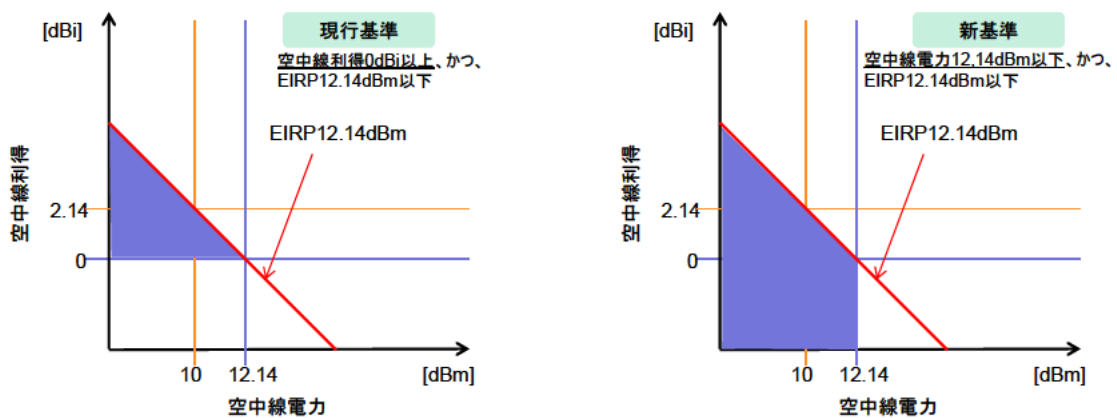
図 3-7 空中線分離時のテレメータ・テレコントロール・データ伝送の空中線利得、空中線電力及び EIRP
