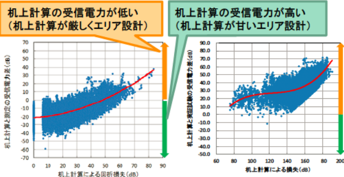
机上計算の回折損失と受信電力差の傾向 (多重回折損失計算) 机上計算の回折損失と受信電力差の傾向 (ITU-R P.1812)
