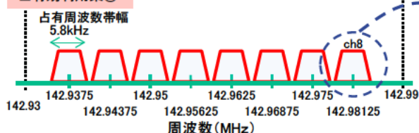
周波数軸上のch配置
