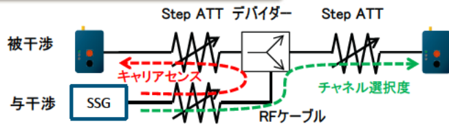
図4-29 測定構成
