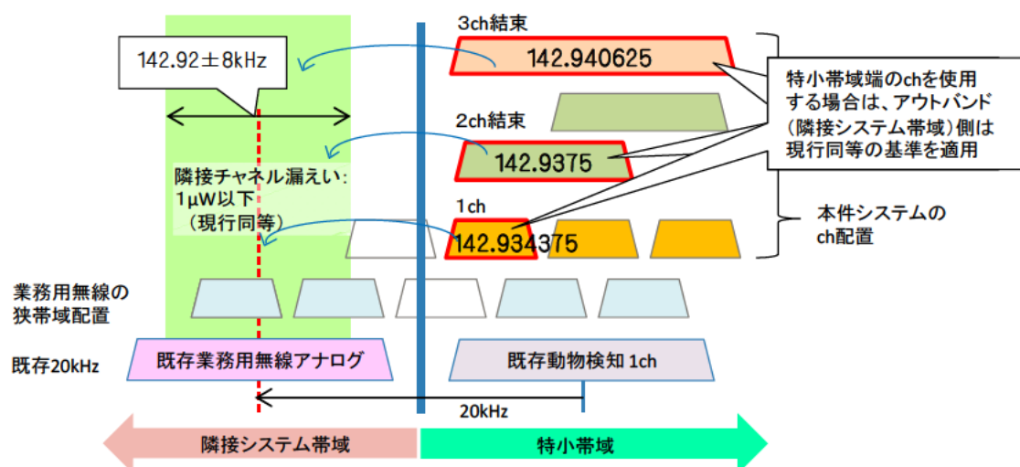
図2-16 隣接システムへの影響を考慮した隣接チャンネル漏えい電力の基準の設定
