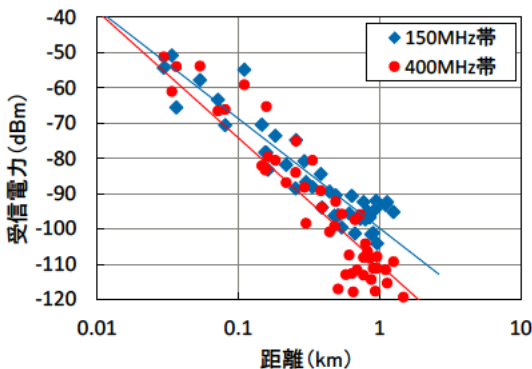
図4-10 受信電力の距離特性
