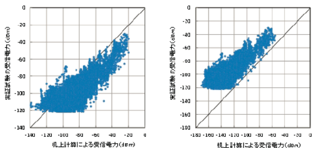
多重回折損失計算との比較 ITU-R P.1812との比較
