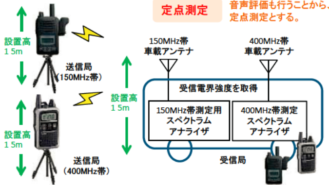
図4-8 測定構成図
