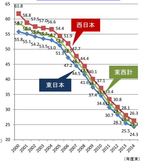
芯線使用率(メタル)の推移
