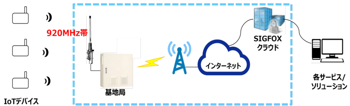
図 10 SIGFOX のネットワーク概要
