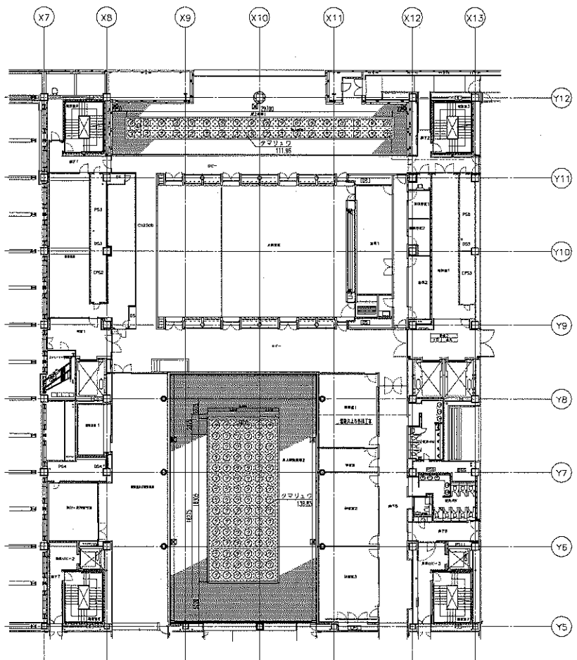
5階上改築(5階)平面図 S=1:200
