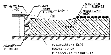
5階上改築断面図 S=1:20
