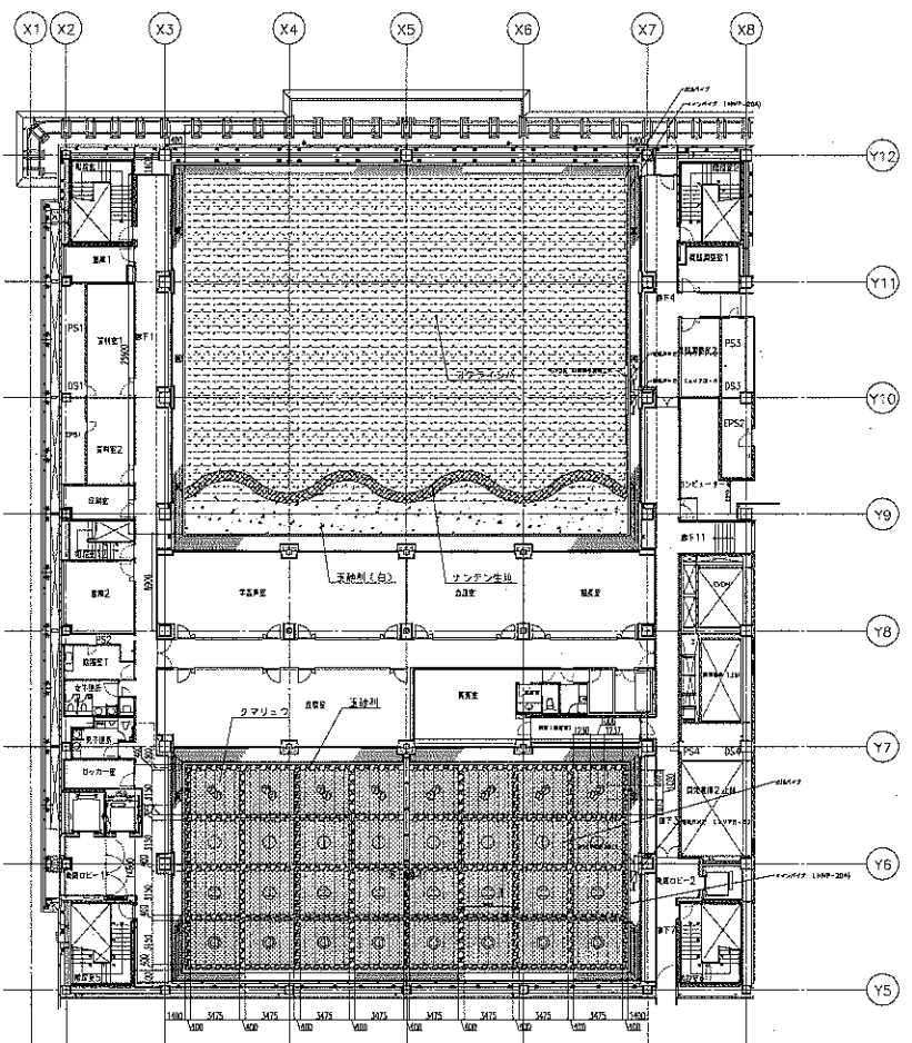
6階上改築(6階)平面図 S=1:200
