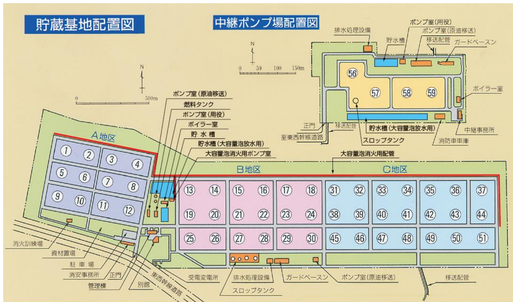
別紙 1-1 施設配置図 (むつ小川原国家石油備蓄基地)
