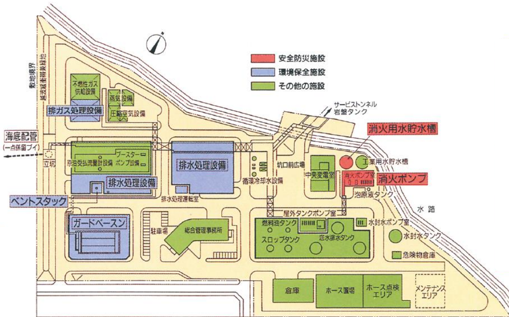
施設配置図 (③串木野国家石油備蓄基地)
