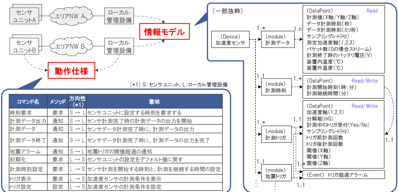
図 II-25 加速度センサの情報モデルの TTC 標準概要
