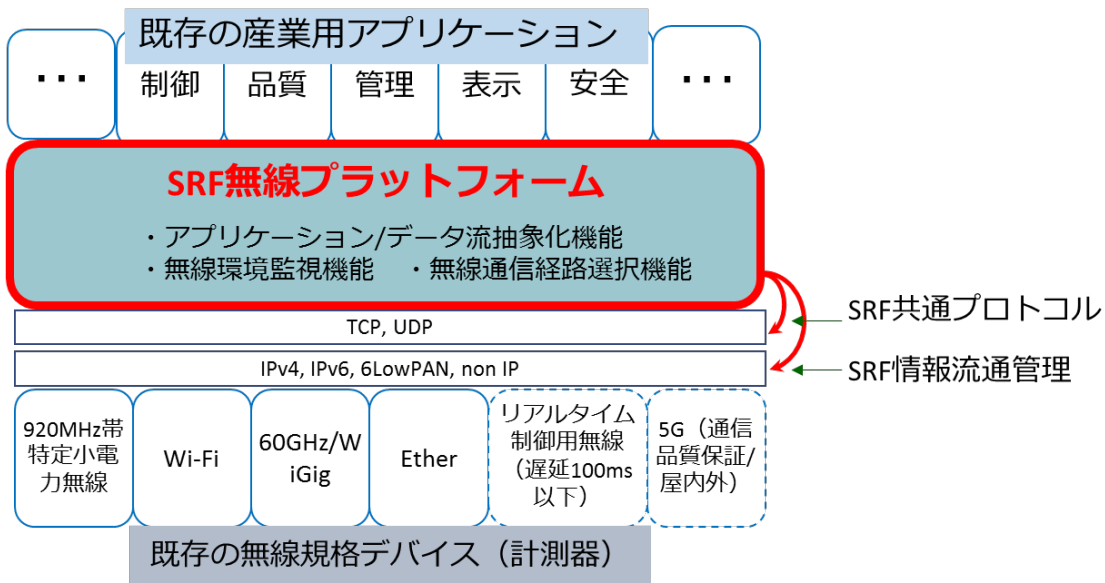
図 II-20 FFPJ の国際標準化に向けた取組内容
