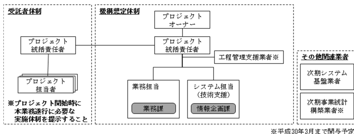
図 6-1 全体体制
