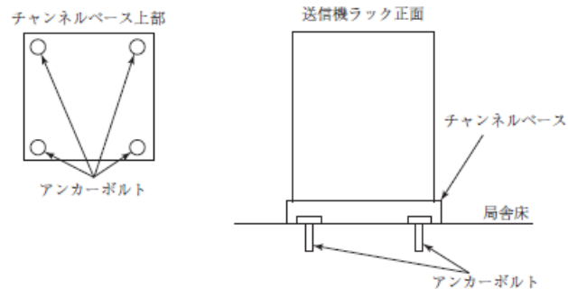
第15図 機器ラックを床に固定する例
