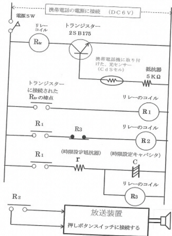
携帯電話機でチャイムを起動させる電気回路図
