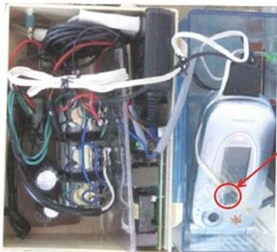
携帯電話機と、光から電気に変換する電気回路
