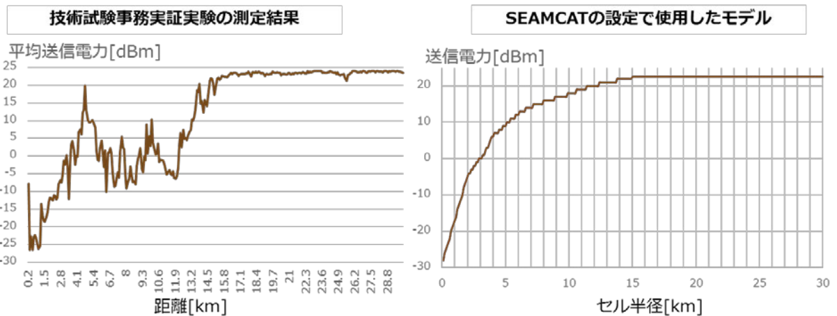
図 3-17 実証実験の測定結果及びモデル化した送信電力分布
