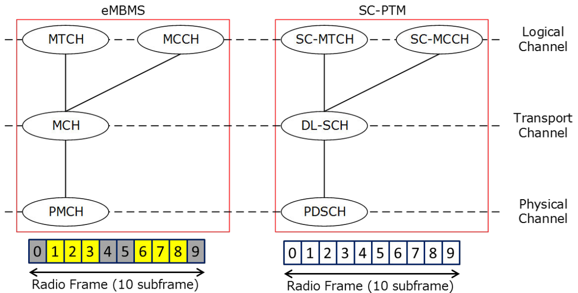
図 4 eMBMS と SC-PTM のチャネルマッピングの比較
