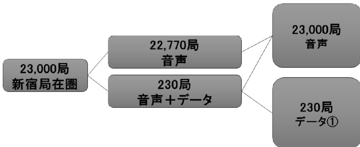
図 3-6 全国 30 万移動局時の新宿局の通信種別ごとの移動局数
