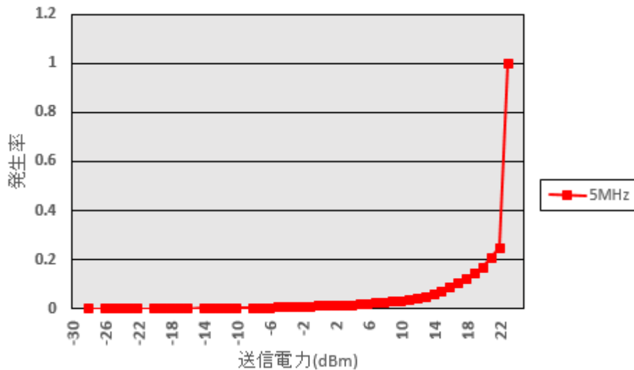
図 3-20 送信電力累積確率モデル C(30km 半径セル)
