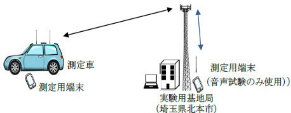
図 3-1 実験構成
