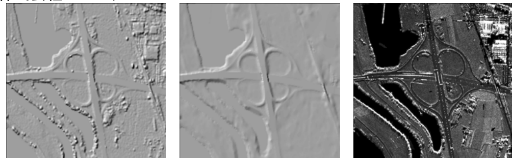
IFSARを用いた地形図作成 (左) DSM (中) DTM (右) オルソ化画像 IFSAR: InterFerometric Synthetic Aperture Radar (出典:INTERMAP社)
