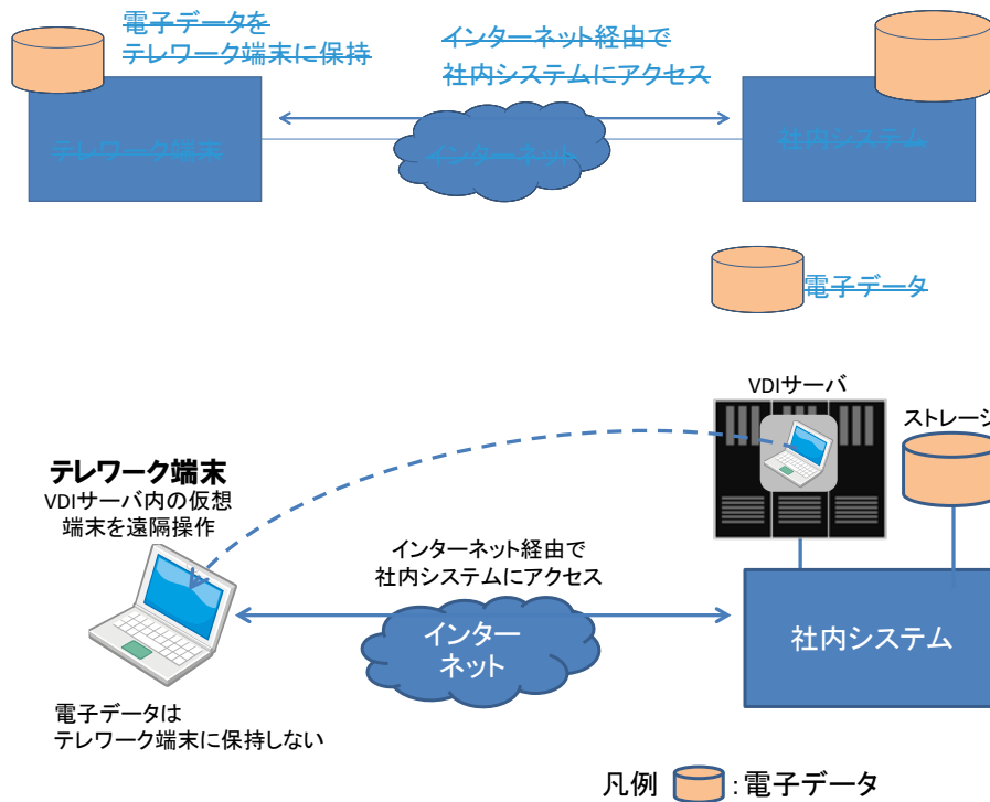
図 4 オンライン持ち出し型仮想デスクトップ方式
