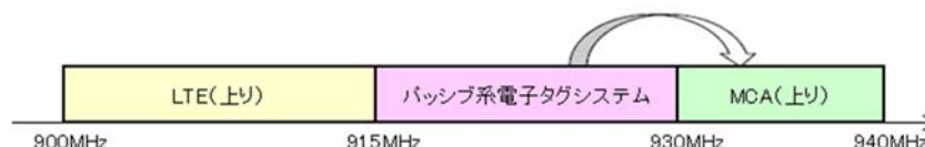
参図 4 - 7 パッシブ系電子タグシステムから MCA 上りへの影響
